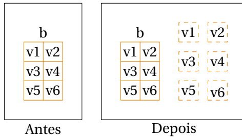
FIGURA 6.1: Área de trabalho antes e depois de attach(b)
