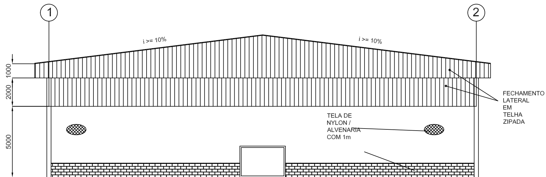
ELEVAÇÃO TRANSVERSAL (EIXO A/EIXO J) MEDIODAS EM mm
