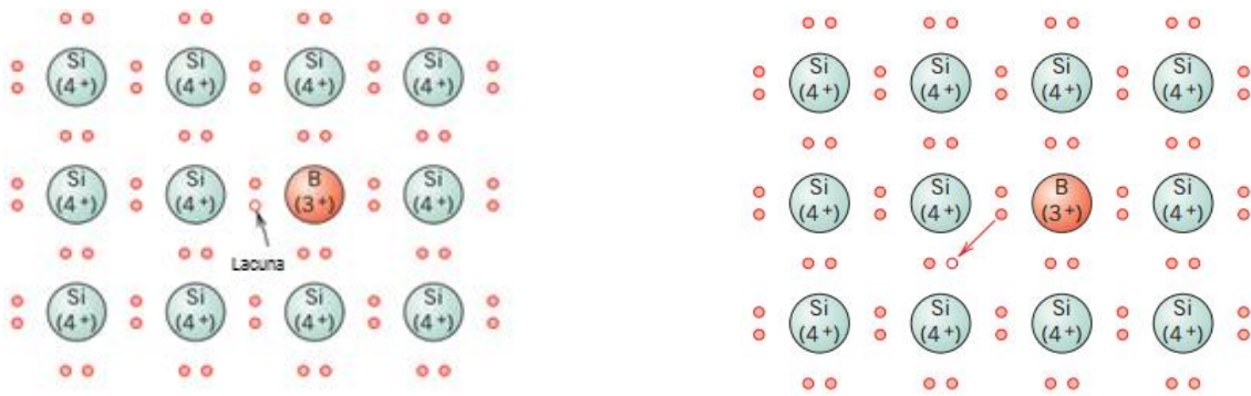
Figura 4b: Condução elétrica em um semiconductor extrínseco do tipo-p
