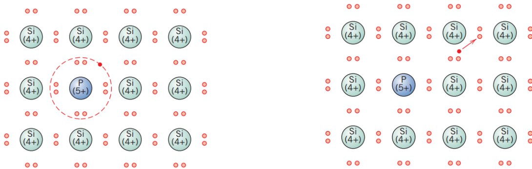
Figura 3b: Condução elétrica em um semiconductor extrínseco do tipo-n
