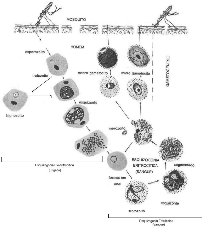
CICLO VITAL DO PLASMODIUM VIVAX
