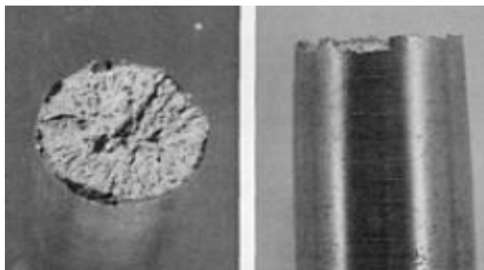
Figura 1 – Fratura de um aço grau X100 (Mirone e Corallo, 2013).
