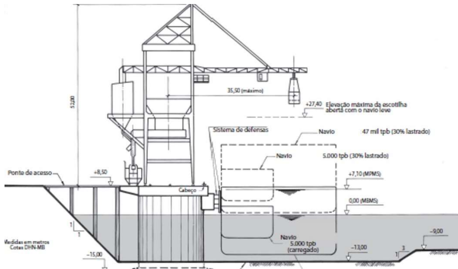
Exemplos de bordas livres de cais em função do tipo de carga movimentada em alguns portos no mundo
