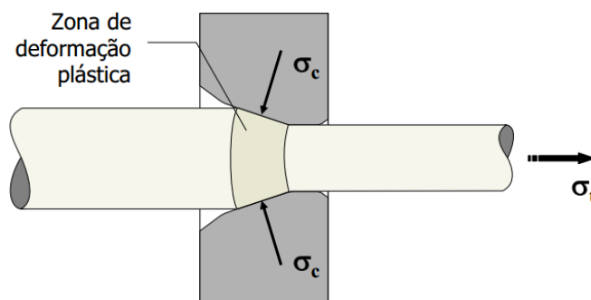
Figura 1.8.9: Mecânica da Trefilação.
