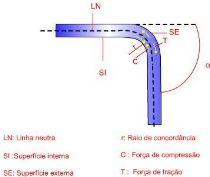
Figura 1.8.3: Esforços e Linha Neutra em Tira submetida a Dobramento.
