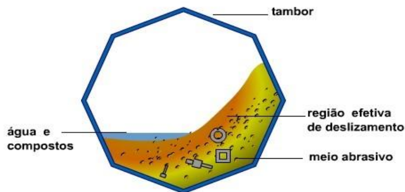
Figura 1.8.1: Representação do processo de tamboreamento.
