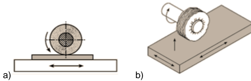
Figura 1.8.2: Processo de polimento. a) vista frontal b) vista isométrica
