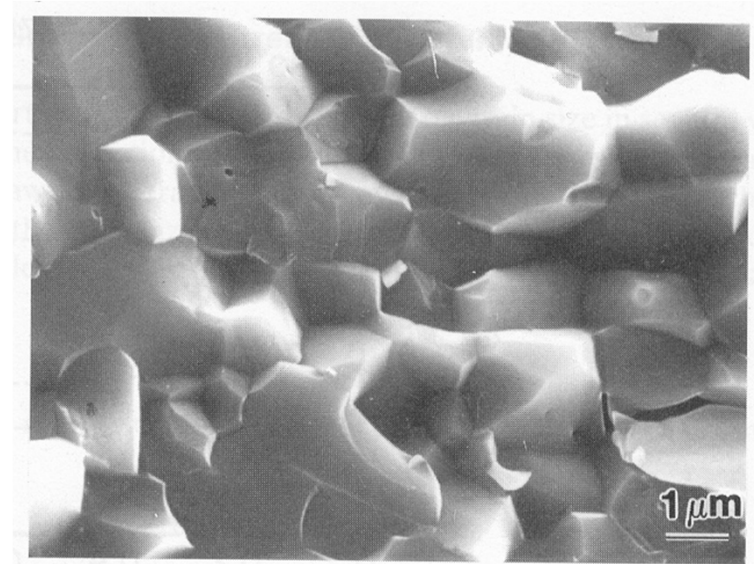
Fratura intergranular em alumina com 99,4% de pureza
