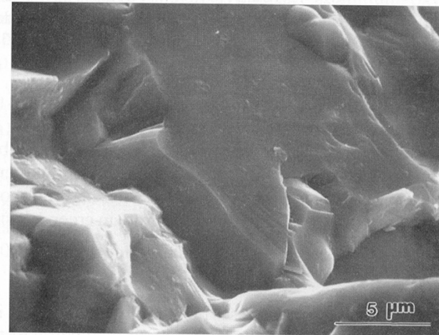
Clivagem em cerâmica (TiB 2 )
