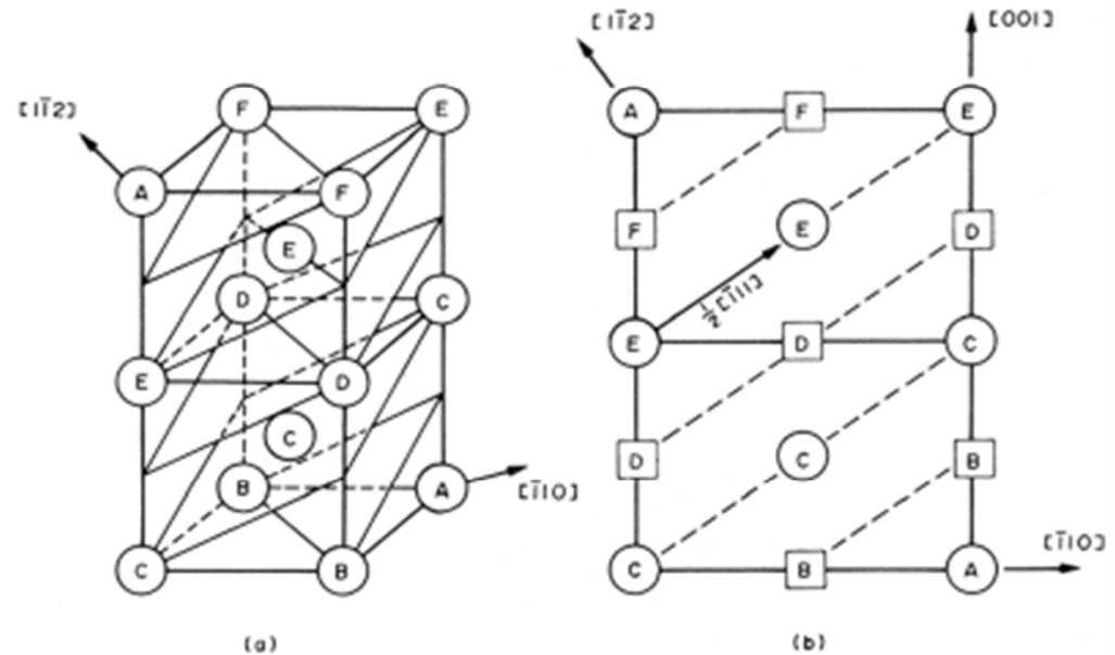
Planos de escorregamento (111) na estrutura CFC
