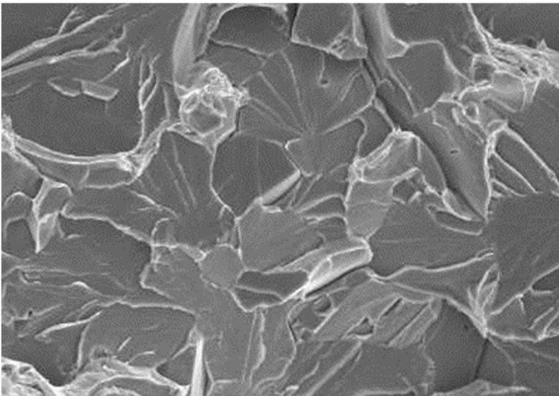
Clivagem em aço frágil
