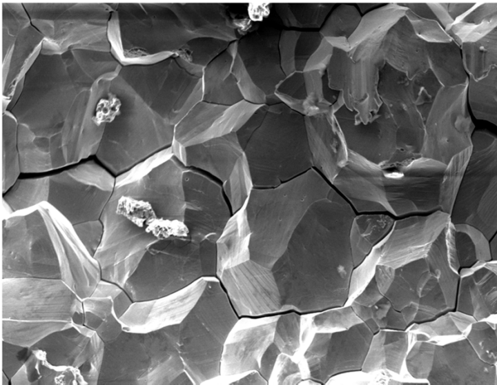
Fratura intergranular em aço
