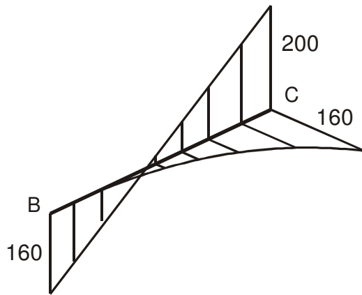
M (kN.m)
