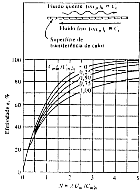
Fig. 11.18 Efetividade num trocador de calor em contracorrente. (De Kays e London [10].)
