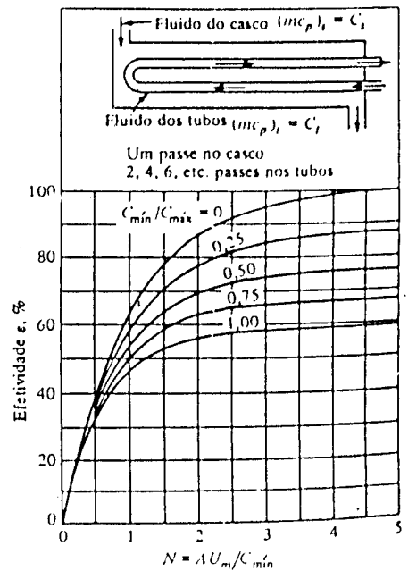
Fig. 11.20 Efetividade num trocador de um passe no casco e dois, quatro, seis, etc. passes nos tubos. (De Kays e London, [10].)
