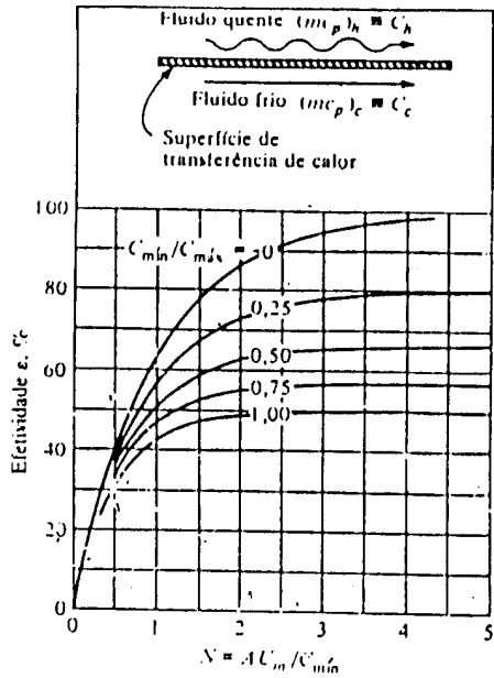
Fig. 11.17 Efetividade num trocador de calor com correntes paralelas. (De Kays e London [10].)
