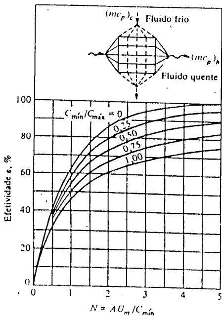
Fig. 11.19 Efetividade num trocador de calor, com correntes cruzadas, ambas não-misturadas. (De Kays e London [10].)
