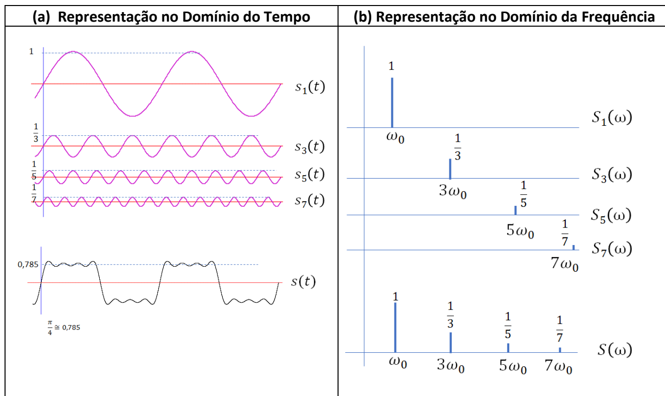
Quadro 2 – Representações de funções trigonométrica no Domínio do Tempo e da Frequência
