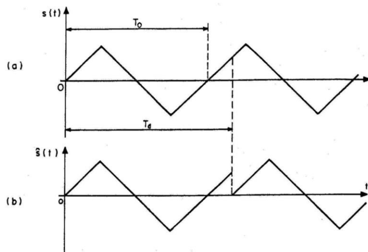
Figura 3 - A origem dos erros de vazamento.
