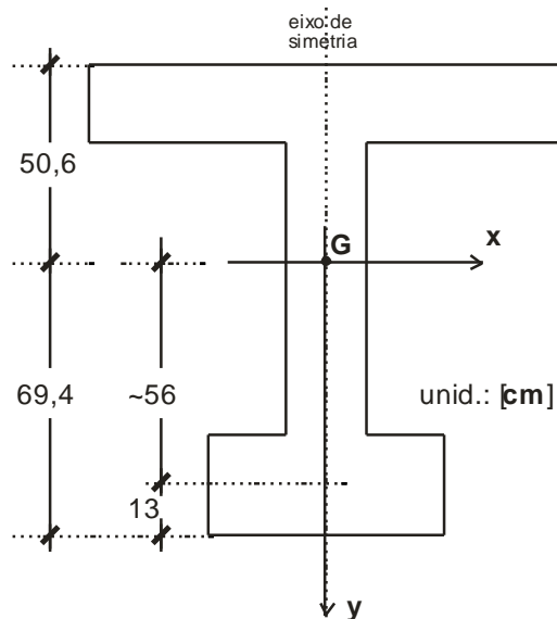
seção transversal
