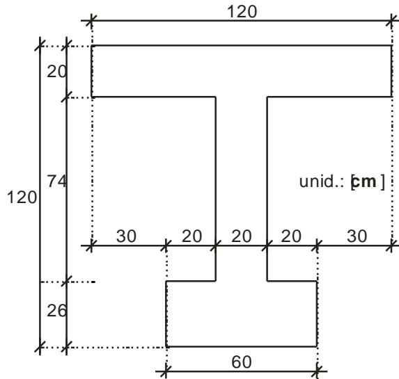
seção transversal
