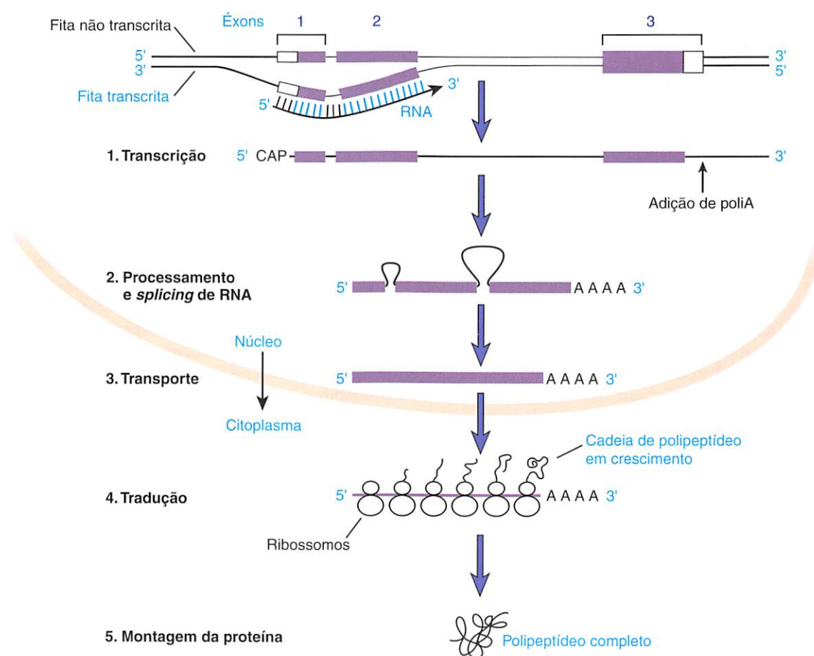
Figura 3-5 Fluxo de informação do DNA até o RNA e até a proteína para um gene hipotético com três éxons e dois íntrons. Dentro dos éxons, a cor roxa indica as sequências codificantes. As etapas incluem transcrição, processamento e splicing de RNA, transporte de RNA do núcleo para o citoplasma, e tradução.
