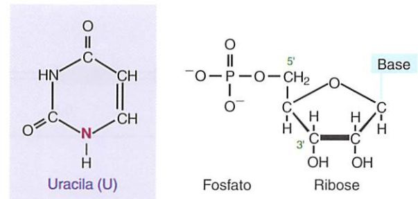
Figura 3-3 A pirimidina uracila e a estrutura de um nucleotídeo no RNA. Observe que o açúcar ribose substitui o açúcar desoxirribose do DNA. Compare com a Figura 2-2.
