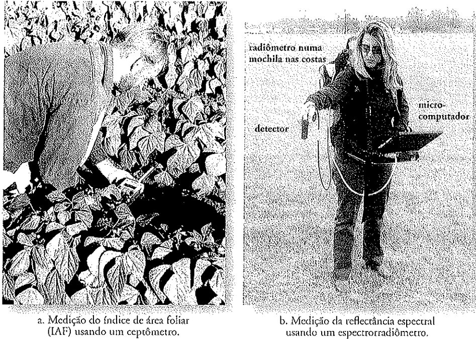
Figura 1-1 Dados in situ (no local) são coletados no campo. a) Um pesquisador está coletando medidas de índice de área foliar (IAF) de soja ( Glycine max L. Merrill) usando um ceptômetro, que mede o número de regiões do substrato que foram iluminadas diretamente sem interceptação pelo dossel vegetal. As medições são feitas bem acima do dossel e no solo, sob o dossel. As medidas de IAF in situ podem ser usadas para calibrar as estimativas de IAF derivadas de dados de sensores remotos. b) Medidas de reflectância espectral de vegetação estão sendo coletadas usando um espectrorradiômetro colocado a aproximadamente 1 m acima do dossel. As medidas de reflectância espectral in situ podem ser usadas para calibrar medidas de reflectância espectral obtidas por um sistema de sensoriamento remoto.
