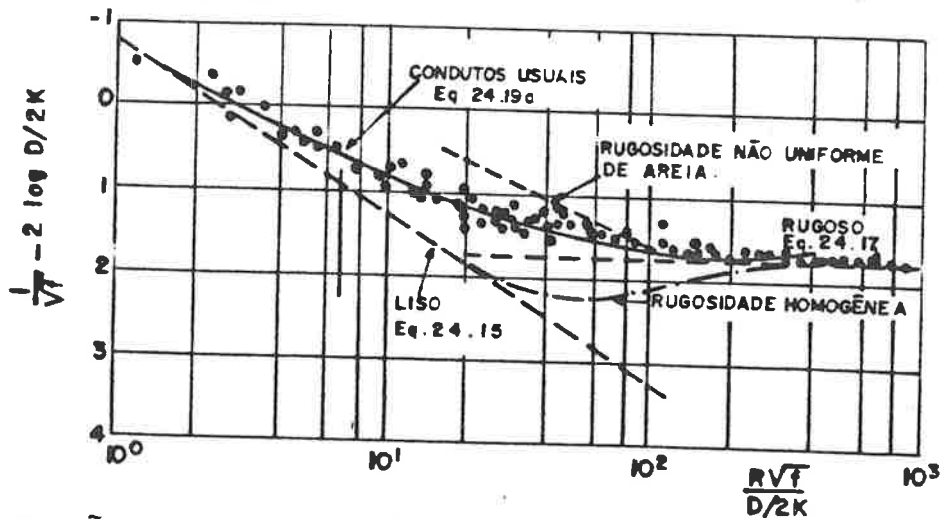
Fig.24.9-Função geral da rugosidade para condutos de rugosidade homogênea e heterogênea.
