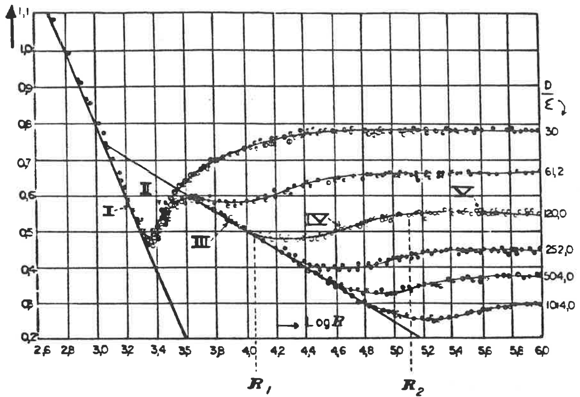
Fig.24.7-Diagrama de Nikuradse.
