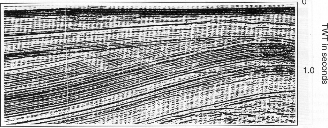
Top lap
