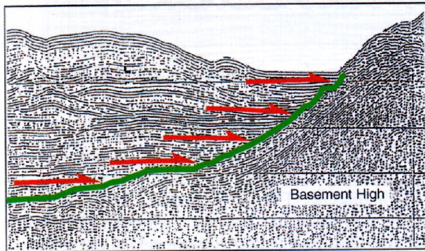
Onlap
