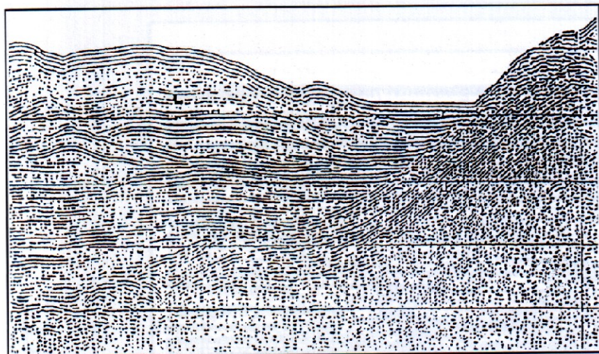
Onlap
