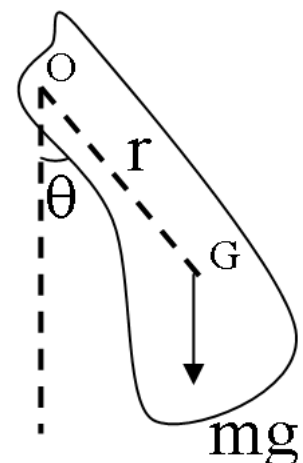
Figura 1. Ilustração do pêndulo composto.
