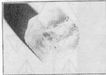
Fig. 3. Sphalerite (011).
