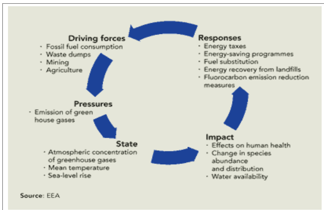
Gráfico 10 MARCO ORDENADOR. AGENCIA AMBIENTAL EUROPEA
