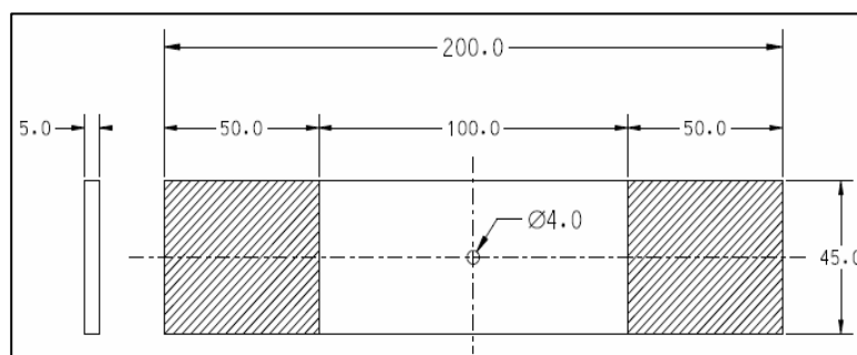
Figura 3 – Geometria e dimensões do corpo de prova, do tipo chapa, utilizado nos ensaios de fadiga, para k_t = 2,76 , dimensão em mm (Bonazzi, 2013).
