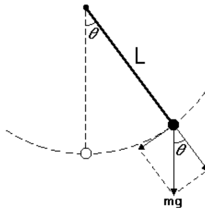
Figura 2.2 - pêndulo simples
