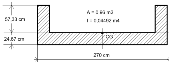
(a) Seção transversal da viga e detalhe.
