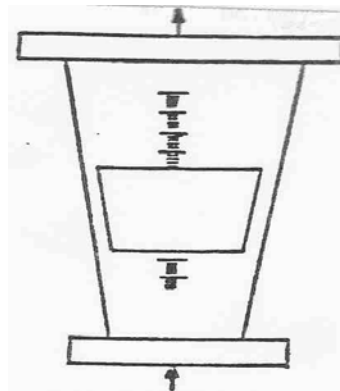
Fig. 1 Esquema do Rotâmetro
