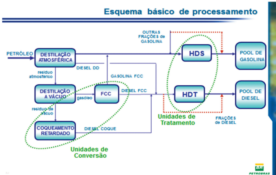
Figura 1 Processo de refino de gasolina e Diesel
