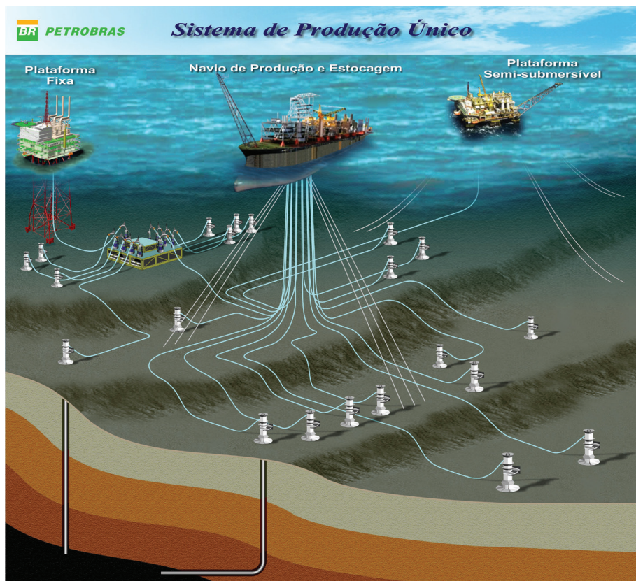
Figura 5 Árvore de natal, manifold e risers em sistema de produção de petróleo offshore
