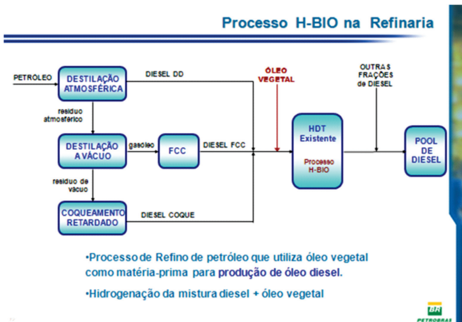
Figura 2 Processo de produção de Diesel H-BIO em refinaria de petróleo
