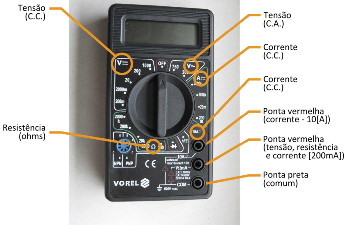
Fig. 4.2 Multímetro.
