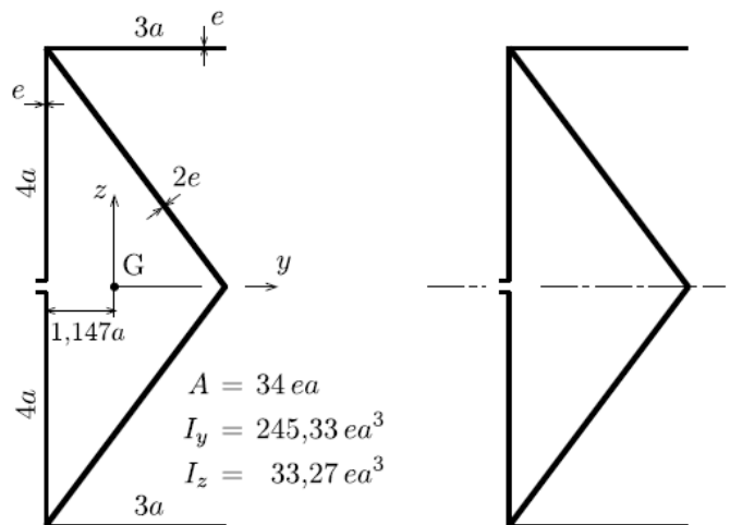
Seção transversal
