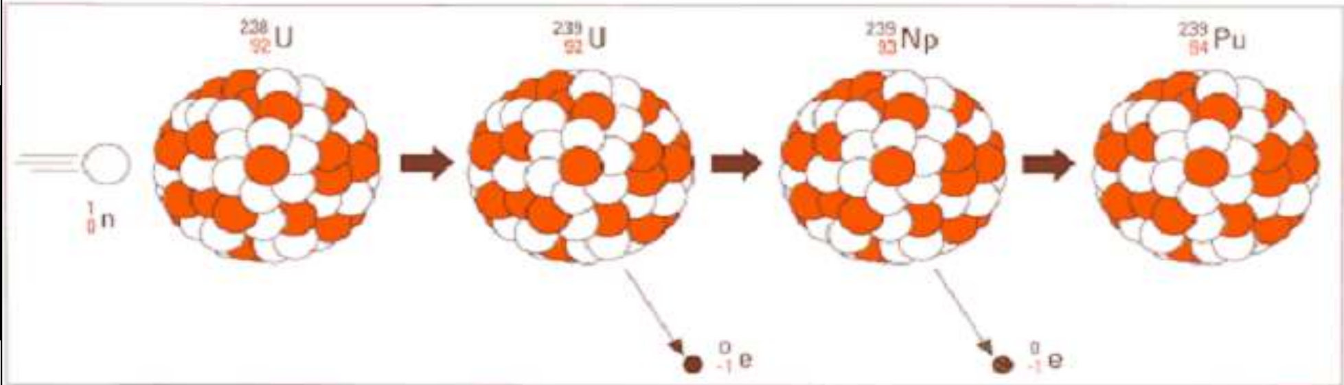
Reação de captura no U-238, produção de Pu-239
