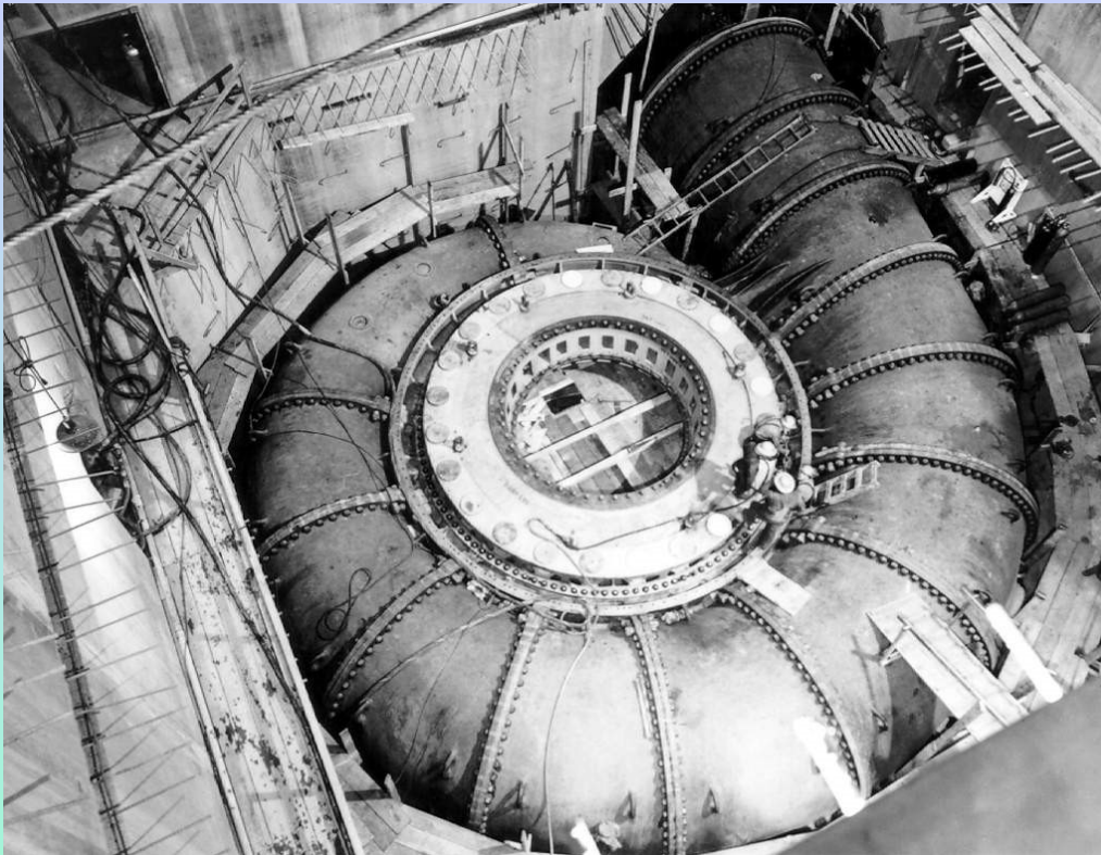
Duto de entrada de uma turbina Francis
