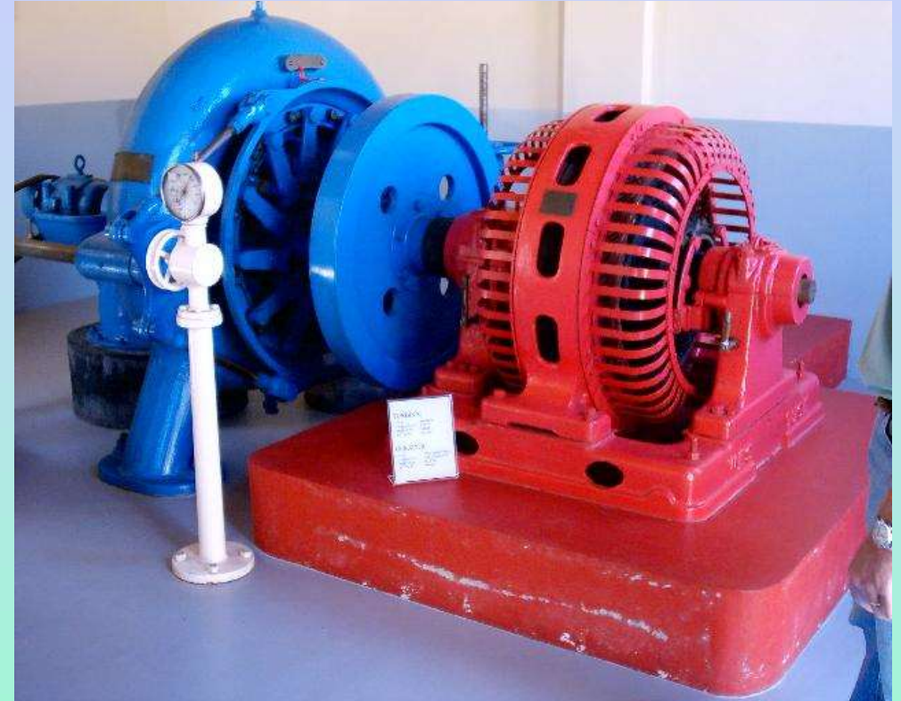
Turbina Francis (azul) e gerador (vermelho) usados na Usina Hidrelétrica de Foz do Areia
