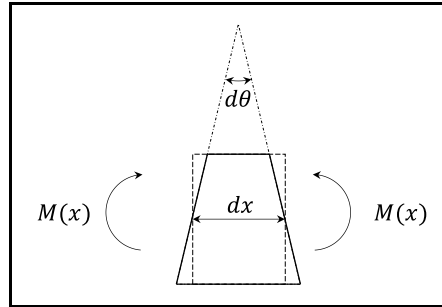
Figura 19 – Elemento de comprimento infinitesimal.
