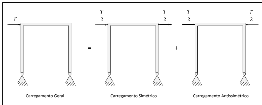
Figura 23 – Decomposição de um carregamento geral em um carregamento simétrico e outro antissimétrico.
