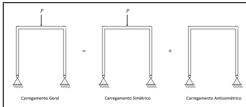
Figura 24 – Decomposição de um carregamento geral em um carregamento simétrico e outro antissimétrico.
