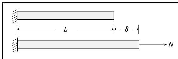
Figura 8 – Barra submetida a uma força axial.
