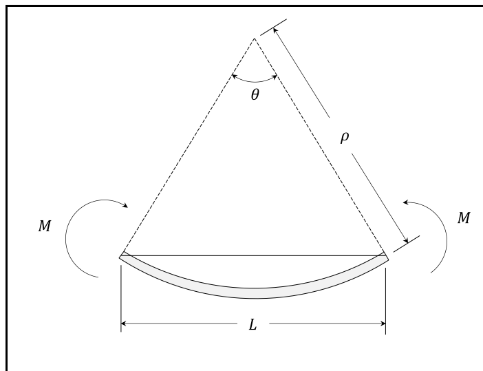
Figura 17 – Barra sob flexão uniforme.
