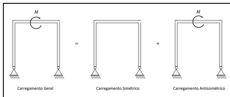
Figura 25 – Decomposição de um carregamento geral em um carregamento simétrico e outro antissimétrico.
