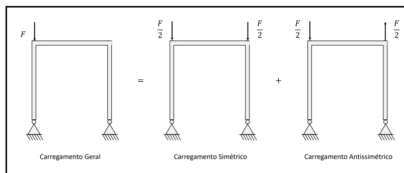
Figura 22 – Decomposição de um carregamento geral em um carregamento simétrico e outro antissimétrico.
