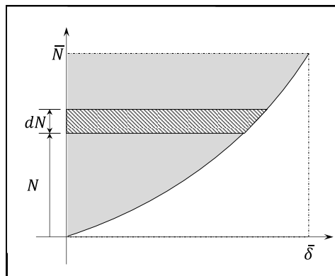
Figura 6 – Cálculo do trabalho complementar.
