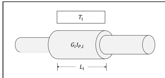
Figura 14 – Eixo escalonado.
