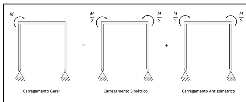
Figura 21 – Decomposição de um carregamento geral em um carregamento simétrico e outro antissimétrico.
