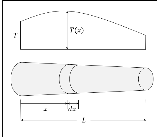
Figura 15 – Eixo não-uniforme.
