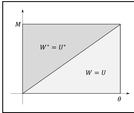
Figura 18 – Energias de deformação e complementar na flexão uniforme.
