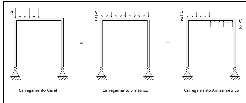
Figura 26 – Decomposição de um carregamento geral em um carregamento simétrico e outro antissimétrico.
