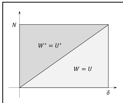
Figura 9 – Material elástico linear.
