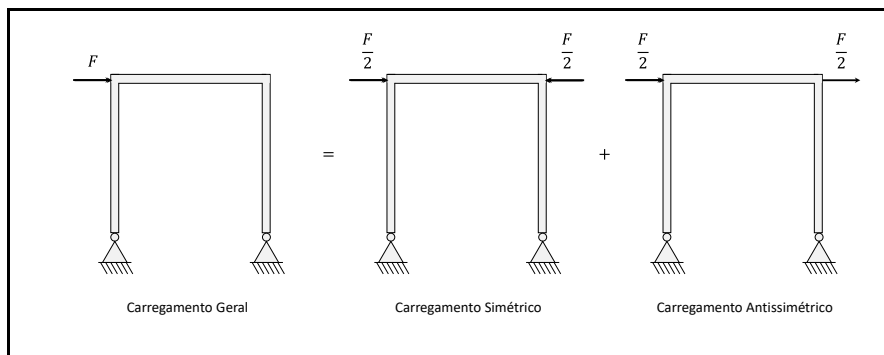
Figura 20 – Decomposição de um carregamento geral em um carregamento simétrico e outro antissimétrico.
