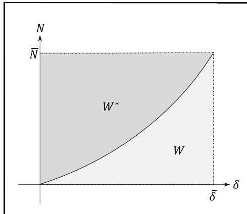
Figura 5 – Trabalho e trabalho complementar.
