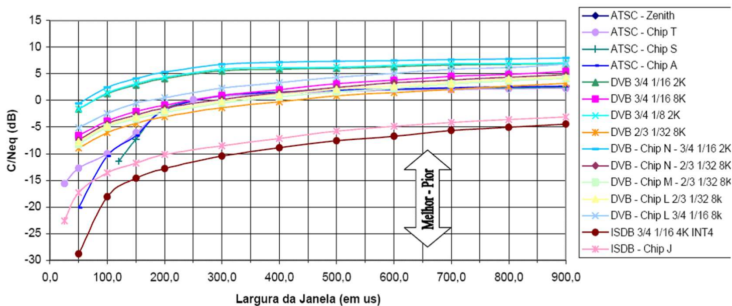
Gráfico 2.5.3.1: Relação entre largura da janela de ruído e relação sinal interferente para ruído impulsivo
