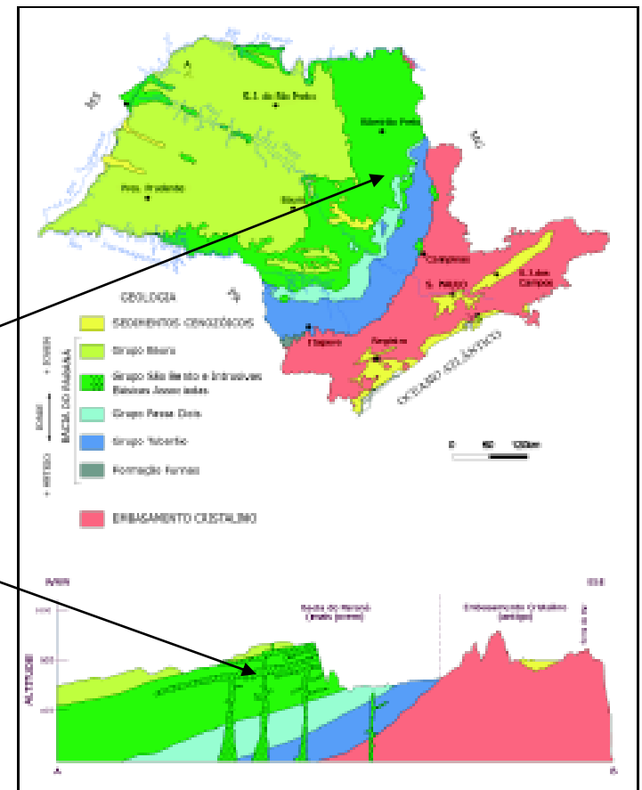
Figura 4 - Distribuição das principais unidades geológicas do Estado de São Paulo
