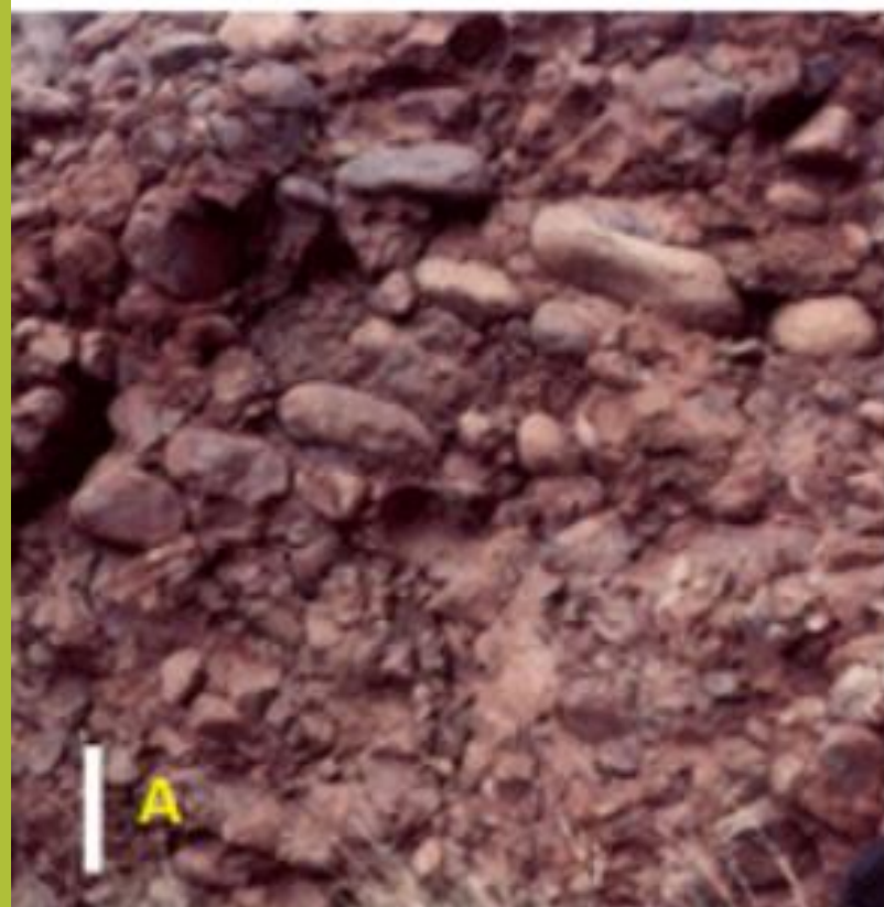
Conglomerado (A) da Formação de Itararé e diamicito (B).
