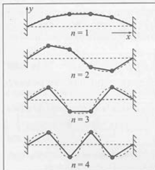
Figura 4.22 — Modos transversais de 4 partículas
