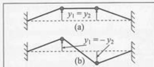
Figura 4.21 — Modos normais
