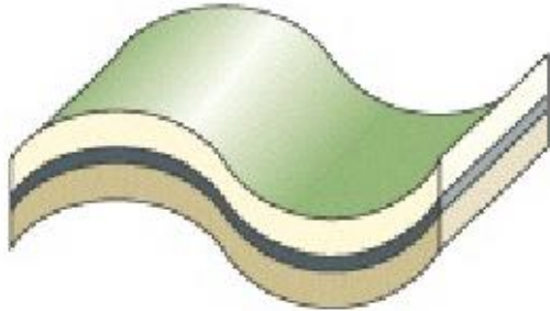
DOBRAMENTO
