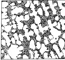
Fig. 59 — Veios de grafita do tipo D. Veios pequenos e curtos agrupados preenchendo o espaço interdendrítico como austenítico. 100 x.
