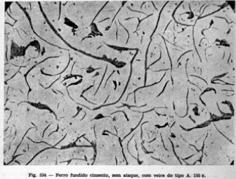
Fig. 54 — Ferro fundido cinzento, sem ataque, com veios do tipo A. 150 x.
