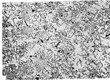
Fig. 56 — Ferro fundido cinzento, sem ataque, com veios do tipo B. 150 x.
