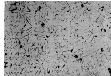
Fig. 542 — Ferro fundido cinzento com grafita do tipo E. 100 x.
