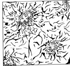
Fig. 55 — Veios de grafita do tipo B. Veios com disposição radial em torno de núcleos de aspecto austenítico. 100 x.
