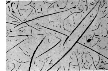
— Ferro fundido cinzento, sem ataque, com veios tipo C. 150 x.
