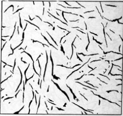
Fig. 53 — Veios de grafita do tipo A. Veios curvos as veios laminadas, com orientação à 45°. 100 x.
