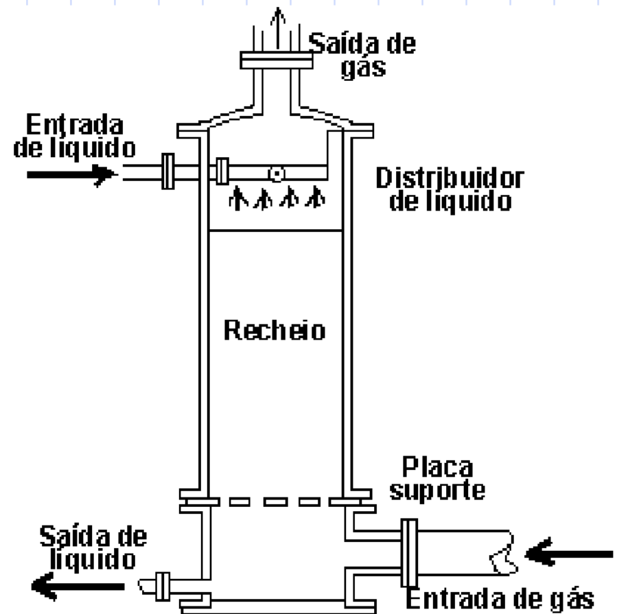
Esquema de uma coluna de enchimento
