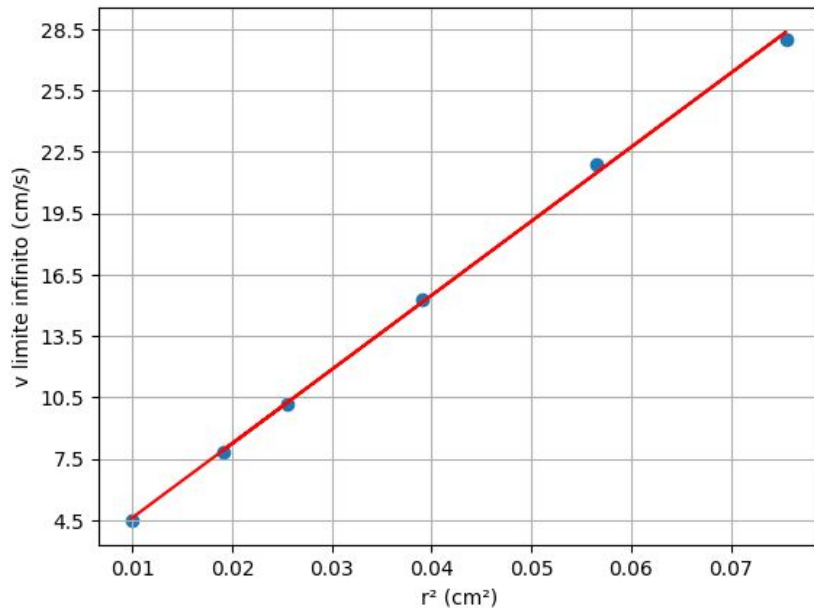
Gráfico Velocidade limite Lubrax25W50
