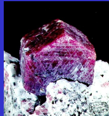
Coríndon
