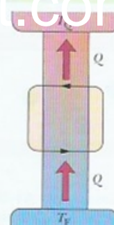
Figura 20-15 Os elementos de um refrigerador perfeito, ou seja, um refrigerador que transfere energia de uma fonte fria para uma fonte quente sem necessidade de trabalho.
