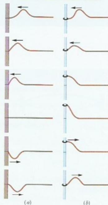
Figura 16-18 (a) Um pulso proveniente da direita é refletido na extremidade esquerda da corda, que está amarrada em uma parede. Note que o pulso refletido sofre uma inversão em relação ao pulso incidente. (b) Neste caso, a extremidade esquerda da corda está amarrada em um anel que pode deslizar sem atrito para cima e para baixo em uma barra e o pulso não é invertido pela reflexão.
