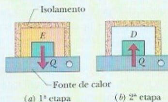
Figura 20-6 Os blocos da Fig. 20-5 podem passar do estado inicial para o estado final de uma forma reversível se usarmos uma fonte de temperatura controlável (a) para extrair calor reversivelmente do bloco E e (b) para adicionar calor reversivelmente ao bloco D .
