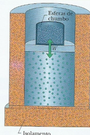
Figura 18-15 Uma expansão adiabática pode ser realizada removendo esferas de chumbo do êmbolo. O processo pode ser invertido a qualquer momento acrescentando novas esferas.
