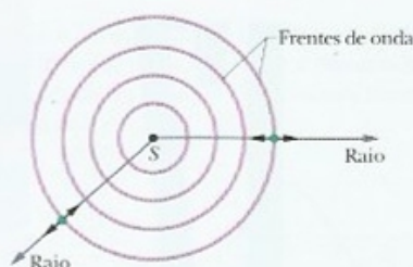
Figura 17-2 Uma onda sonora se propaga a partir de uma fonte pontual S em um meio tridimensional. As frentes de onda formam esferas com centro em S ; os raios são perpendiculares às frentes de onda. As setas de duas cabeças mostram que os elementos do meio oscilam paralelamente aos raios.
