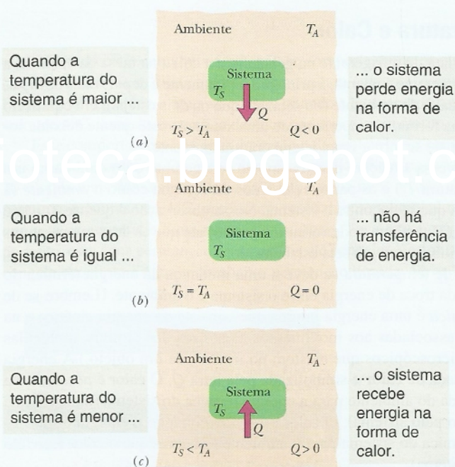
Figura 18-12 Se a temperatura de um sistema é maior que a temperatura ambiente, como em (a), uma certa quantidade Q de calor é perdida pelo sistema para o ambiente para que o equilíbrio térmico (b) seja restabelecido. (c) Se a temperatura do sistema é menor que a temperatura ambiente, uma certa quantidade de calor é absorvida pelo sistema para que o equilíbrio térmico seja restabelecido.
