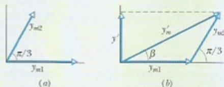
Figura 16-15 (a) Dois fasores de módulos y_{m1} e y_{m2} com uma diferença de fase de \pi/3 . (b) A soma vetorial dos fasores em qualquer instante fornece o módulo y'_m do fasor da onda resultante.
