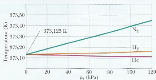
Figura 18-6 Temperaturas medidas por um termômetro de gás a volume constante, com o bulbo imerso em água fervente. Para calcular a temperatura usando a Eq. 18-5, a pressão p_3 foi medida no ponto triplo da água. Três gases diferentes no bulbo do termômetro fornecem resultados diferentes para diferentes pressões do gás, mas quando a quantidade de gás é reduzida (o que diminui o valor de p_3 ), as três curvas convergem para 373,125 K.
