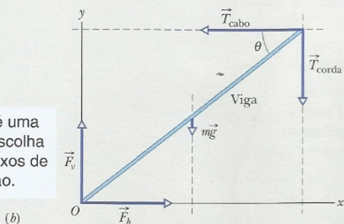
Figura 12-6 (a) Um cofre está pendurado em uma lança de guindaste composta por uma viga uniforme e um cabo de aço horizontal. (b) Diagrama de corpo livre da viga.
