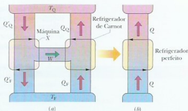
Figura 20-16 (a) A máquina térmica X alimenta um refrigerador de Carnot. (b) Se, como alega o inventor, a máquina X é mais eficiente que a máquina de Carnot, a combinação mostrada em (a) é equivalente ao refrigerador perfeito mostrado em (b). Como isso viola a segunda lei da termodinâmica, concluímos que a máquina X não pode ser mais eficiente que uma máquina de Carnot.
