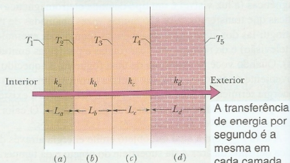
Figura 18-22 Uma parede de quatro camadas através da qual existe transferência de calor.
