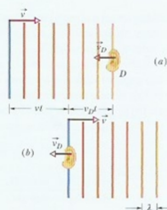
Figura 17-20 Frentes de onda que se deslocam para a direita (a) alcançam e (b) passam pelo detector D , que se move no sentido oposto. No intervalo de tempo t , as frentes de onda percorrem uma distância vt para a direita e D percorre uma distância v_D t para a esquerda.
