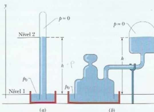
Figura 14-5 (a) Um barômetro de mercúrio. (b) Outro barômetro de mercúrio. A distância h é a mesma nos dois casos.
