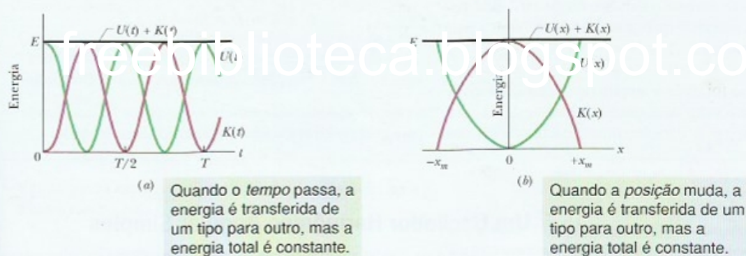
Figura 15-6 (a) Energia potencial U(t) , energia cinética K(t) e energia mecânica E em função do tempo t para um oscilador harmônico linear. Observe que todas as energias são positivas e que a energia potencial e a energia cinética passam por dois máximos em cada período. (b) Energia potencial U(x) , energia cinética K(x) e energia mecânica E em função da posição x para um oscilador harmônico linear de amplitude x_m . Para x = 0 , a energia é toda cinética; para x = \pm x_m , é toda potencial.
