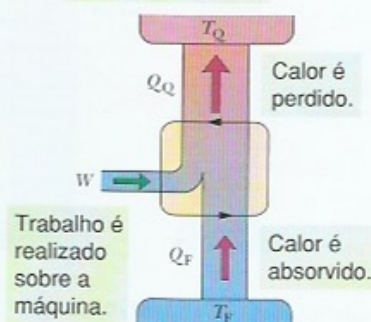
Figura 20-14 Os elementos de um refrigerador. As duas setas pretas horizontais no centro representam uma substância de trabalho operando ciclicamente, como em um diagrama p - V . Uma energia Q_F é transferida em forma de calor da fonte fria, que está à temperatura T_F , para a substância de trabalho; uma energia Q_Q é transferida em forma de calor da substância de trabalho para a fonte quente, que está à temperatura T_Q . Um trabalho W é realizado sobre o refrigerador (na realidade, sobre a substância de trabalho) pelo ambiente.
