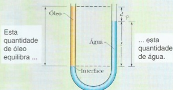
Figura 14-4 O óleo do lado esquerdo fica mais alto que a água do lado direito porque a massa específica do óleo é menor que a da água. As duas colunas de fluido produzem a mesma pressão p_{\text{int}} na interface.
