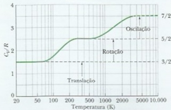
Figura 19-14 Curva de C_V/R em função da temperatura para o hidrogênio (um gás diatômico). Como existe uma energia mínima para as rotações e oscilações, apenas as translações são possíveis em temperaturas muito baixas. Quando a temperatura aumenta, começam as rotações. As oscilações começam em temperaturas ainda maiores.
