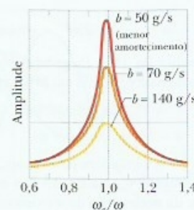
Figura 15-16 A amplitude do deslocamento x_m de um oscilador forçado varia quando a frequência angular \omega_e da força externa varia. As curvas da figura correspondem a três valores diferentes da constante de amortecimento b .
