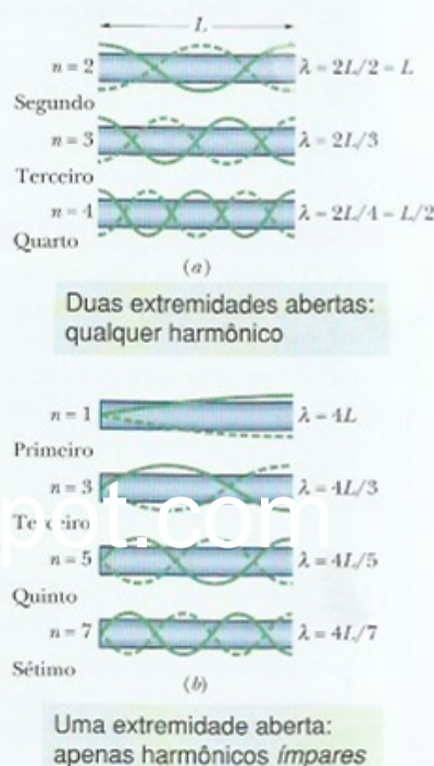
Figura 17-14 Ondas estacionárias em tubos, representadas por curvas de pressão em função da posição. (a) Com as duas extremidades do tubo abertas, qualquer harmônico pode ser produzido no tubo. (b) Com uma extremidade aberta, apenas os harmônicos ímpares podem ser produzidos.
