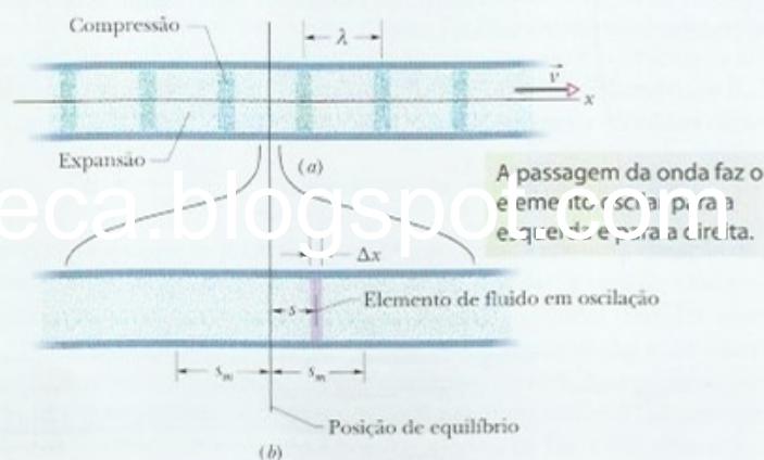
Figura 17-4 (a) Uma onda sonora que se propaga com velocidade v em tubo longo cheio de ar é composta por uma série de expansões e compressões periódicas do ar que se deslocam ao longo do tubo. A onda é mostrada em um instante arbitrário. (b) Uma vista horizontal ampliada de uma pequena parte do tubo. Quando a onda passa, um elemento de ar de espessura \Delta x oscila para a esquerda e para a direita em um movimento harmônico simples em torno da posição de equilíbrio. No instante mostrado em (b), o elemento se encontra deslocado de uma distância s para a direita da posição de equilíbrio. O deslocamento máximo, para a direita ou para a esquerda, é s_m .
