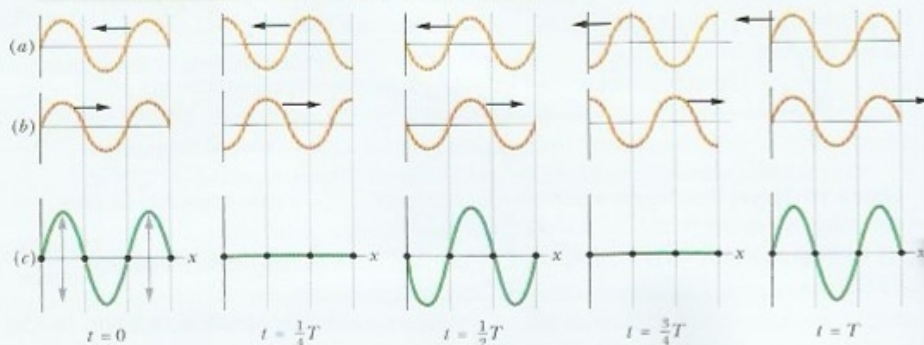
Figura 16-16 (a) Cinco instantâneos de uma onda se propagando para a esquerda, em instantes t indicados abaixo da parte (c) ( T é o período das oscilações). (b) Cinco instantâneos de uma onda igual à de (a), mas se propagando para a direita, nos mesmos instantes t . (c) Instantâneos correspondentes para a superposição das duas ondas na mesma corda. Nos instantes t = 0, T/2 e T , a interferência é totalmente construtiva, ou seja, os picos se alinham com picos e os vales com vales. Em t = T/4 e 3T/4 , a interferência é totalmente destrutiva, pois os picos se alinham com vales. Alguns pontos (os nós, indicados por pontos) permanecem imóveis; outros (os antinós) oscilam com amplitude máxima.
