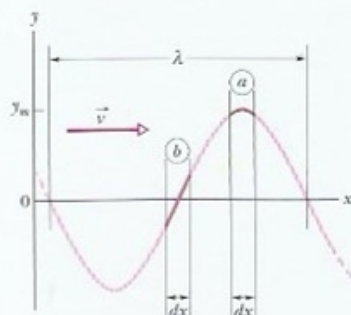
Figura 16-9 Instantâneo de uma onda progressiva em uma corda no instante t = 0 . O elemento a da corda está sofrendo um deslocamento y = y_m e o elemento b está sofrendo um deslocamento y = 0 . A energia cinética depende da velocidade transversal do elemento; a energia potencial, do alongamento.
