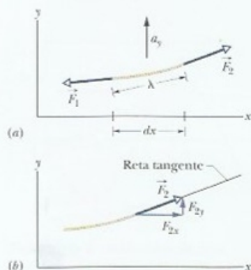
Figura 16-10 (a) Um elemento da corda quando uma onda senoidal transversal se propaga em uma corda esticada. As forças \vec{F}_1 e \vec{F}_2 agem nas extremidades do elemento, produzindo uma aceleração \vec{a} com uma componente vertical a_y . (b) A força na extremidade direita do elemento está dirigida ao longo de uma reta tangente ao lado direito do elemento.
