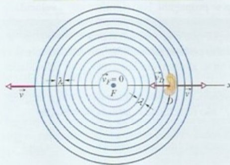
Figura 17-18 Uma fonte sonora estacionária F emite frentes de onda esféricas, mostradas com uma separação de um comprimento de onda, que se expandem radialmente com velocidade v . Um detector D , representado por uma orelha, se move com velocidade v_D em direção à fonte. O detector mede uma frequência maior por causa do movimento.
