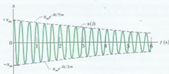
Figura 15-15 A função deslocamento x(t) do oscilador amortecido da Fig. 15-14. A amplitude, que é dada por x_m e^{-bt/2m} , diminui exponencialmente com o tempo.
