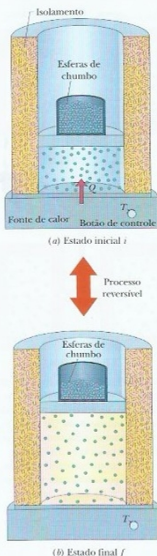
Figura 20-3 Expansão isotérmica de um gás ideal, realizada de forma reversível. O gás possui o mesmo estado inicial i e o mesmo estado final f que no processo irreversível da Fig. 20-1. A Eq. 20-2
