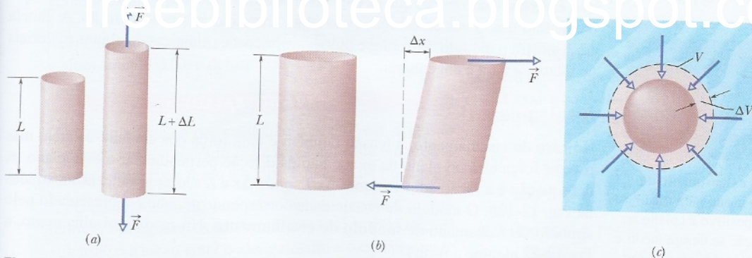
Figura 12-10 (a) Um cilindro submetido a uma tensão trativa sofre um alongamento \Delta L . (b) Um cilindro submetido a uma tensão de cisalhamento sofre uma deformação \Delta x , semelhante à de uma pilha de cartas de baralho. (c) Uma esfera maciça submetida a uma tensão hidrostática uniforme aplicada por um fluido tem o volume reduzido de um valor \Delta V . Todas as deformações mostradas estão muito exageradas.
