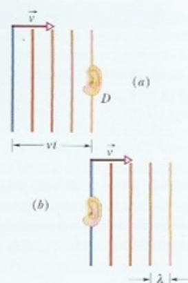
Figura 17-19 As frentes de onda da Fig. 17-18, supostas planas, (a) alcançam e (b) passam por um detector estacionário D ; elas percorrem uma distância vt para a direita no intervalo de tempo t .
