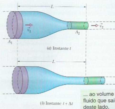
Figura 14-15 Um fluido escoa da esquerda para a direita com vazão constante através de um segmento de tubo de comprimento L . A velocidade do fluido é v_1 no lado esquerdo e v_2 no lado direito. A área de seção reta é A_1 no lado esquerdo e A_2 no lado direito. Do instante t em (a) até o instante t + \Delta t em (b), a quantidade de fluido mostrada em cor violeta entra do lado esquerdo e uma quantidade igual, mostrada em cor verde, sai do lado direito.
