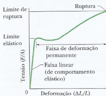
Figura 12-12 Curva tensão-deformação de um corpo de prova de aço como o da Fig. 12-11. O corpo de prova sofre uma deformação permanente quando a tensão atinge o limite elástico e se rompe quando a tensão atinge o limite de ruptura do material.
