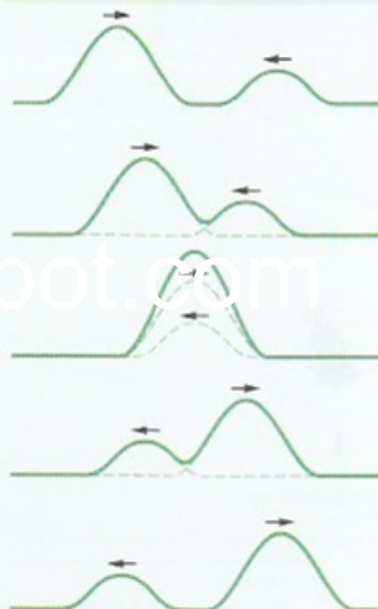
Figura 16-11 Uma série de instantâneos que mostra dois pulsos se propagando em sentidos opostos em uma corda esticada. O princípio da superposição se aplica quando os pulsos passam um pelo outro.
