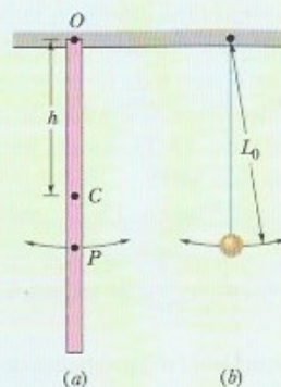
Figura 15-11 (a) Uma régua de um metro suspensa por uma das extremidades para formar um pêndulo físico. (b) Um pêndulo simples cujo comprimento L_0 é escolhido para que os períodos dos dois pêndulos sejam iguais. O ponto P do pêndulo (a) é o centro de oscilação.
