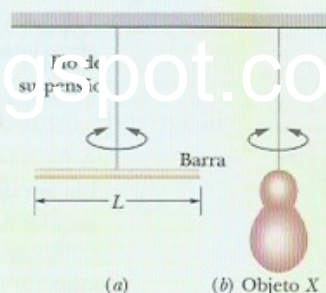
Figura 15-8 Dois pêndulos de torção, compostos (a) por um fio e uma barra e (b) pelo mesmo fio e um objeto de forma irregular.
