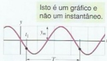
Figura 16-5 Gráfico do deslocamento do elemento da corda situado em x = 0 em função do tempo, quando a onda senoidal da Fig. 16-4 passa pelo elemento. A amplitude y_m está indicada. Um período T típico, medido a partir de um tempo arbitrário t_1 , também está indicado.
