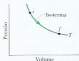
Figura 20-4 Diagrama p - V para a expansão isotérmica reversível da Fig. 20-3. Os estados intermediários, que são agora estados de equilíbrio, estão indicados por uma curva.
