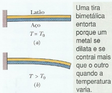
Figura 18-10 (a) Uma tira bimetálica, formada por uma tira de latão e uma tira de aço soldadas, à temperatura T_0 . (b) Quando a temperatura é maior que a temperatura de referência, a tira se enverga para baixo, como na figura. Quando a temperatura é maior que a temperatura de referência, a tira se enverga para cima. Muitos termostatos funcionam com base nesse princípio, fazendo ou desfazendo um contato elétrico de acordo com a temperatura em que se encontram.
