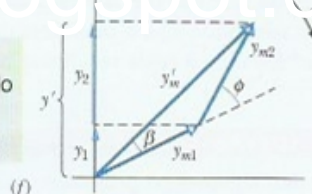
Figura 16-14 (a)–(d) Um fasor de módulo y_{m1} girando em torno de uma origem com velocidade angular \omega representa uma onda senoidal. A projeção y_1 do fasor no eixo vertical representa o deslocamento de um ponto pelo qual a onda passa. (e) Um segundo fasor, também de velocidade angular \omega , mas de módulo y_{m2} e girando com um ângulo \phi constante de diferença em relação ao primeiro fasor, representa uma segunda onda, com uma constante de fase \phi . (f) A onda resultante é representada pelo vetor soma dos dois fasores, y'_m .
