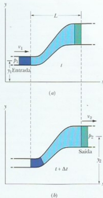
Figura 14-19 Um fluido escoou com vazão constante através de um comprimento L de um tubo, da extremidade de entrada, à esquerda, até a extremidade de saída, à direita. Do instante t em (a) ao instante t + \Delta t em (b), uma quantidade de fluido, representada na cor violeta, entra pela extremidade esquerda e uma quantidade igual, representada na cor verde, sai pela extremidade direita.
