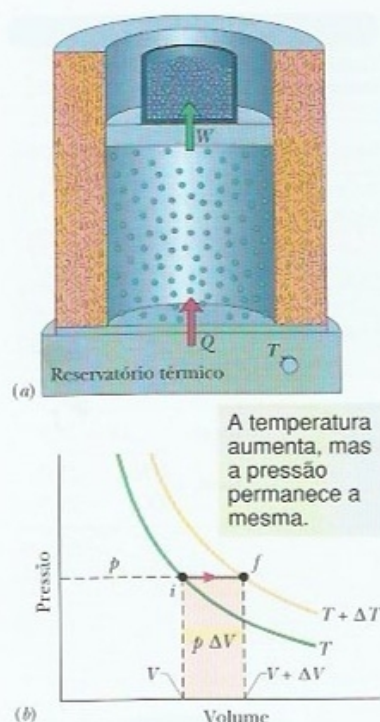
Figura 19-11 (a) A temperatura de um gás ideal é aumentada de T para T + \Delta T em um processo à pressão constante. É adicionado calor e é realizado trabalho para levantar o êmbolo. (b) O processo em um diagrama p - V . O trabalho p\Delta V é dado pela área sombreada.
