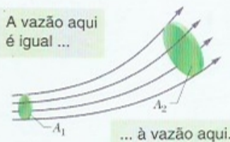
Figura 14-17 Um tubo de fluxo é definido pelas linhas de fluxo que o envolvem. A vazão é a mesma em todas as seções retas de um tubo de fluxo.
