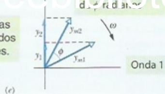
Figura 16-14 (a)–(d) Um fasor de módulo y_{m1} girando em torno de uma origem com velocidade angular \omega representa uma onda senoidal. A projeção y_1 do fasor no eixo vertical representa o deslocamento de um ponto pelo qual a onda passa. (e) Um segundo fasor, também de velocidade angular \omega , mas de módulo y_{m2} e girando com um ângulo \phi constante de diferença em relação ao primeiro fasor, representa uma segunda onda, com uma constante de fase \phi . (f) A onda resultante é representada pelo vetor soma dos dois fasores, y'_m .
