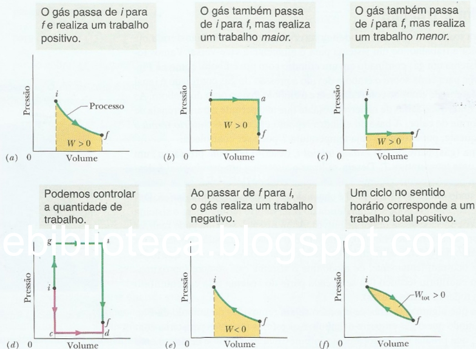
Figura 18-14 (a) A área sombreada representa o trabalho W realizado por um sistema ao passar de um estado inicial i para um estado final f . O trabalho W é positivo porque o volume do sistema aumenta. (b) W continua a ser positivo, mas agora é maior. (c) W continua a ser positivo, mas agora é menor. (d) W pode ser ainda menor (trajetória icdf ) ou ainda maior (trajetória ighf ). (e) Neste caso, o sistema vai do estado f para o estado i quando o gás é comprimido por uma força externa e o volume diminui; o trabalho W realizado pelo sistema é negativo. (f) O trabalho total W_{\text{tot}} realizado pelo sistema durante um ciclo completo é representado pela área sombreada.
