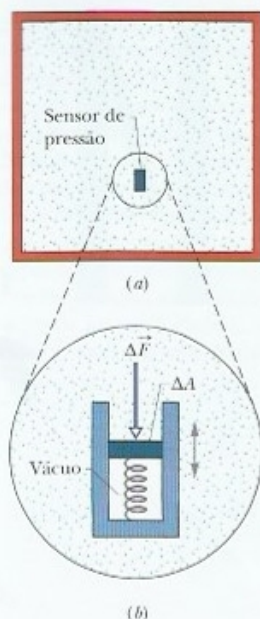
Figura 14-1 (a) Um recipiente cheio de fluido com um pequeno sensor de pressão, mostrado em (b). A pressão é medida pela posição relativa do êmbolo móvel.
