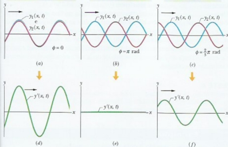
Figura 16-13 Duas ondas senoidais iguais, y_1(x, t) e y_2(x, t) , se propagam em uma corda no sentido positivo de um eixo x . Elas interferem para produzir uma onda resultante y'(x, t) , que é a onda observada na corda. A diferença de fase \phi entre as duas ondas é (a) 0 rad ou 0^\circ , (b) \pi rad ou 180^\circ e (c) 2\pi/3 rad ou 120^\circ . As ondas resultantes correspondentes são mostradas em (d), (e) e (f).
