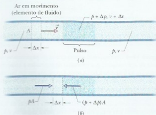
Figura 17-3 Um pulso de compressão se propaga da direita para a esquerda em um tubo longo cheio de ar. O referencial da figura foi escolhido de tal forma que o pulso permanece em repouso e o ar se move da esquerda para a direita. (a) Um elemento de ar de largura \Delta x se move em direção ao pulso com velocidade v . (b) A borda dianteira do elemento penetra no pulso. São mostradas as forças (associadas à pressão do ar) que agem sobre as bordas dianteira e traseira.
