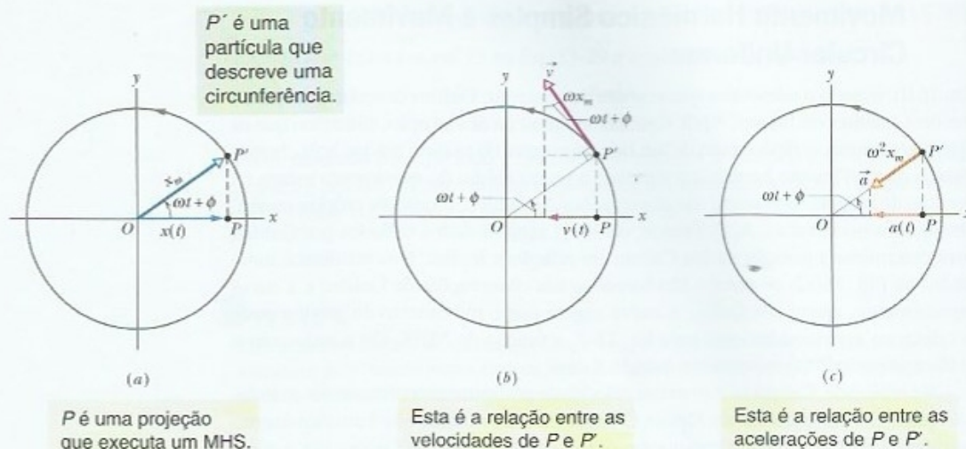
Figura 15-13 (a) Uma partícula de referência P' descrevendo um movimento circular uniforme em uma circunferência de raio x_m . A projeção P da posição da partícula no eixo x executa um movimento harmônico simples. (b) A projeção da velocidade \vec{v} da partícula de referência é a velocidade do MHS. (c) A projeção da aceleração radial \vec{a} da partícula de referência é a aceleração do MHS.
