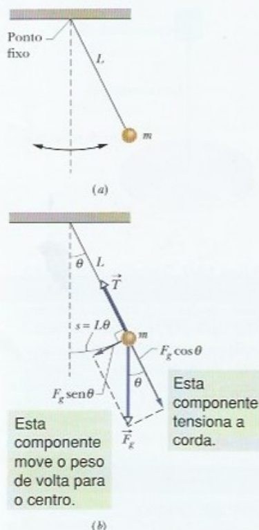
Figura 15-9 (a) Um pêndulo simples. (b) As forças que agem sobre o peso são a força gravitacional \vec{F}_g e a tensão \vec{T} do fio. A componente tangencial F_g \sin \theta da força gravitacional é a força restauradora que tende a levar o pêndulo de volta para a posição central.
