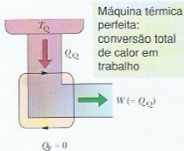
Figura 20-11 Os elementos de uma máquina térmica perfeita, ou seja, uma máquina que converte calor Q_Q de uma fonte quente em trabalho W com 100% de eficiência.
