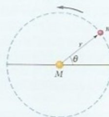
Figura 13-14 Um planeta de massa m girando em torno do Sol em uma órbita circular de raio r .
