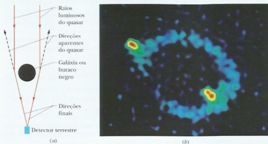
Figura 13-19 (a) A trajetória da luz de um quasar distante se encurva ao passar por uma galáxia ou buraco negro porque a massa da galáxia ou do buraco negro encurva o espaço próximo. Quando a luz é detectada, parece ter sido produzida em um ponto situado no prolongamento da trajetória final (retas tracejadas). (b) Imagem do anel de Einstein conhecido como NGC 4551, obtida pelo projeto de telescópio Arecibo. A fonte de luz (na verdade, ondas de rádio, que são uma forma invisível de luz) está muito atrás da grande galáxia invisível responsável pela formação do anel; uma parte da fonte aparece como dois pontos luminosos no anel. (Cortesia do National Radio Astronomy Observatory)
