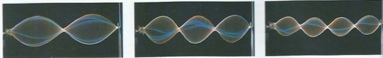
Figura 16-19 Fotografias estroboscópicas revelam ondas estacionárias (imperfeitas) em uma corda excitada por um oscilador na extremidade esquerda. As ondas estacionárias se formam apenas para certas frequências de oscilação. (Richard Megna/Fundamental Photographs)
