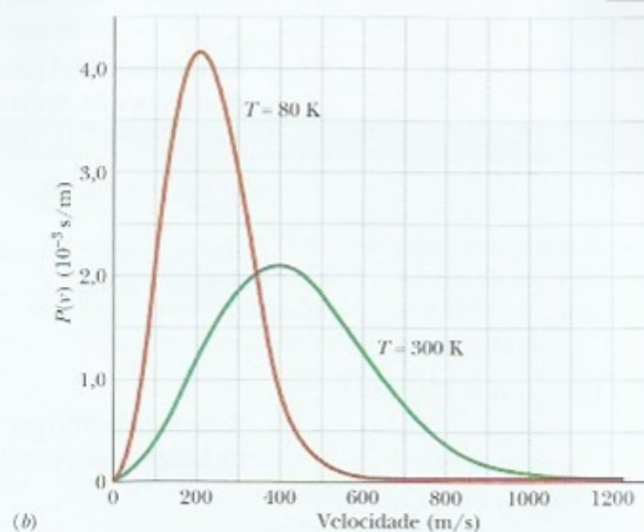
Figura 19-8 (a) A distribuição de velocidades de Maxwell para moléculas de oxigênio a uma temperatura T = 300 K. As três velocidades características estão indicadas. (b) A distribuição de velocidades para 300 K e 80 K. Note que as moléculas se movem mais devagar quando a temperatura é menor. Como se trata de distribuições de probabilidade, a área sob cada curva é igual à unidade.
