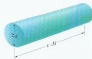
Figura 19-7 No intervalo de tempo \Delta t , a molécula em movimento varre um cilindro de comprimento v\Delta t e raio d .
