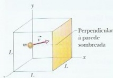
Figura 19-4 Uma caixa cúbica de aresta L contendo n mols de um gás ideal. Uma molécula de massa m e velocidade \vec{v} está prestes a colidir com a parede sombreada de área L^2 . É mostrada também uma reta perpendicular a essa parede.
