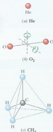
Figura 19-13 Modelos de moléculas usados na teoria cinética dos gases: (a) hélio, uma molécula monoatômica típica; (b) oxigênio, uma molécula diatômica típica; (c) metano, uma molécula poliatômica típica. As esferas representam átomos e os segmentos de reta representam ligações químicas. Dois eixos de rotação são mostrados para a molécula de oxigênio.
