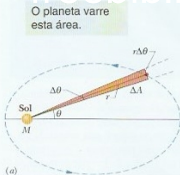
Figura 13-13 (a) No instante \Delta t , o segmento de reta r que liga o planeta ao Sol se desloca de um ângulo \Delta\theta , varrendo uma área \Delta A (sombreada). (b) O momento linear \vec{p} do planeta e suas componentes.
