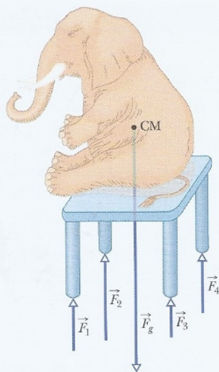
Figura 12-8 A mesa é uma estrutura indeterminada. As quatro forças a que as pernas da mesa estão sujeitas diferem em módulo e não podem ser calculadas usando apenas as leis do equilíbrio estático.
