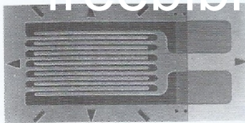
Figura 12-13 Um extensômetro de 9,8 mm por 4,6 mm usado para medir deformações. O dispositivo é colado no corpo cuja deformação se deseja medir e sofre a mesma deformação que o corpo. A resistência elétrica do extensômetro varia com a deformação, permitindo que deformações de até 3% sejam medidas. (Cortesia da Vishay Micro-Measurements Group, Raleigh, NC)
