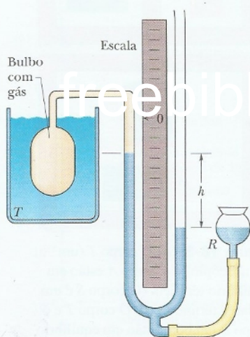
Figura 18-5 Um termômetro de gás a volume constante, com o bulbo imerso em um líquido cuja temperatura T se pretende medir.
