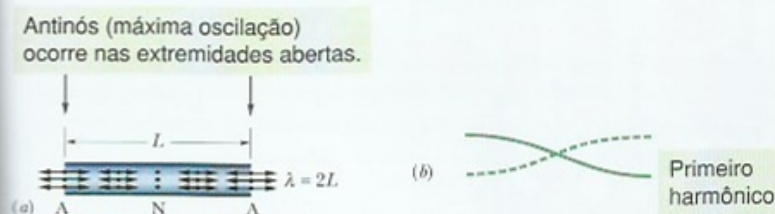
Figura 17-13 (a) O padrão de deslocamento mais simples para uma onda sonora (longitudinal) estacionária em um tubo com as duas extremidades abertas possui um antinó (A) em cada extremidade e um nó (N) no ponto médio do tubo. (Os deslocamentos longitudinais, representados pelas setas duplas, estão muito exagerados.) (b) O padrão correspondente para uma onda transversal em uma corda.
