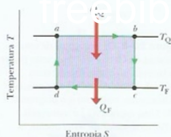
Figura 20-10 O ciclo de Carnot da Fig. 20-9 mostrado em um diagrama temperatura-entropia. Durante os processos ab e cd , a temperatura permanece constante. Durante os processos bc e da , a entropia permanece constante.
