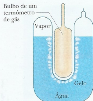
Figura 18-4 Uma célula de ponto triplo, na qual gelo (sólido), água (líquido) e vapor (gás) estão em equilíbrio térmico. Por acordo internacional, a temperatura desta mistura foi definida como 273,16 K. O bulbo de um termômetro de gás a volume constante é mostrado no centro da célula.
