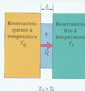
Figura 18-18 Condução de calor. A energia é transferida na forma de calor de um reservatório à temperatura T_Q para um reservatório mais frio à temperatura T_F através de uma placa de espessura L e condutividade térmica k .
