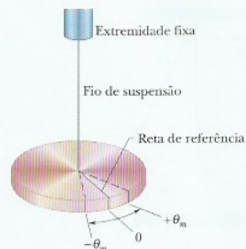
Figura 15-7 O pêndulo de torção é a versão angular do oscilador harmônico linear simples. O disco oscila em um plano horizontal; a reta de referência oscila com amplitude angular \theta_m . A torção do fio de suspensão armazena energia potencial de forma semelhante a uma mola e produz o torque restaurador.
