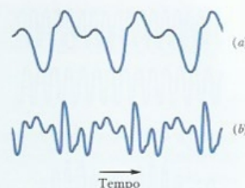
Figura 17-16 Formas de onda produzidas (a) por uma flauta e (b) por um oboé quando uma nota com a mesma frequência fundamental é tocada nos dois instrumentos.
