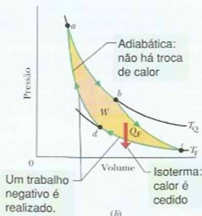
Figura 20-9 Diagrama pressão-volume do ciclo seguido pela substância de trabalho da máquina de Carnot da Fig. 20-8. O ciclo é formado por duas isothermas ( ab e cd ) e duas adiabáticas ( bc e da ). A área sombreada limitada pelo ciclo é igual ao trabalho W por ciclo realizado pela máquina de Carnot.
