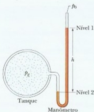
Figura 14-6 Um manômetro de tubo aberto, usado para medir a pressão manométrica do gás contido no tanque da esquerda. O lado direito do tubo é aberto para a atmosfera.
