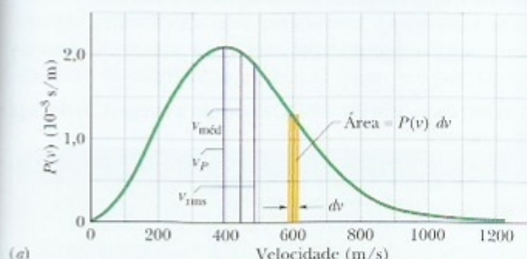
Figura 19-8 (a) A distribuição de velocidades de Maxwell para moléculas de oxigênio a uma temperatura T = 300 K. As três velocidades características estão indicadas. (b) A distribuição de velocidades para 300 K e 80 K. Note que as moléculas se movem mais devagar quando a temperatura é menor. Como se trata de distribuições de probabilidade, a área sob cada curva é igual à unidade.
