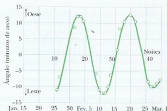
Figura 15-12 O ângulo entre Júpiter e o satélite Calisto do ponto de vista da Terra. Os pontos se baseiam nas observações de Galileu em 1610 e a curva representa um ajuste aos dados, que sugere um movimento harmônico simples. Para a distância média entre Júpiter e a Terra, 10 minutos de arco correspondem a cerca de 2 \times 10^6 km. (Adaptado de A. P. French, Newtonian Mechanics , W.W. Norton & Company, New York, 1971, p. 288.)
