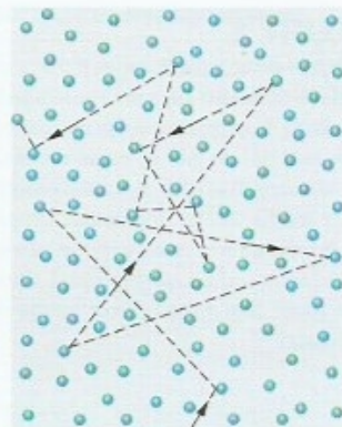
Figura 19-5 Uma molécula se movendo no interior de um gás e colidindo com outras moléculas. Embora as outras moléculas sejam mostradas como se estivessem paradas, também estão se movendo de forma semelhante.
