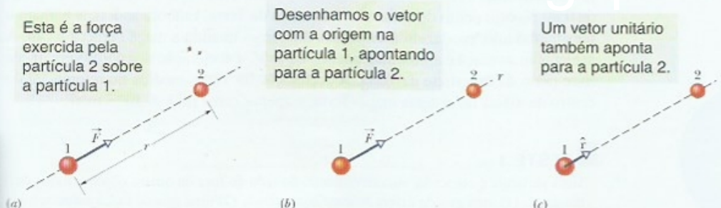
Figura 13-2 (a) A força gravitacional \vec{F} que a partícula 2 exerce sobre a partícula 1 é uma força atrativa porque aponta para a partícula 2. (b) A força \vec{F} está sobre um eixo radial r que passa pelas duas partículas. (c) A força \vec{F} tem o mesmo sentido que o vetor unitário \hat{r} do eixo r .
