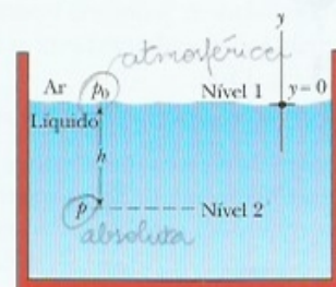
Figura 14-3 A pressão p aumenta com a profundidade h abaixo da superfície do líquido de acordo com a Eq. 14-8.
