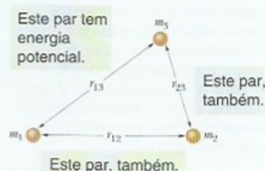
Figura 13-8 Um sistema formado por três partículas. A energia potencial gravitacional do sistema é a soma das energias potenciais gravitacionais dos três pares de partículas.
