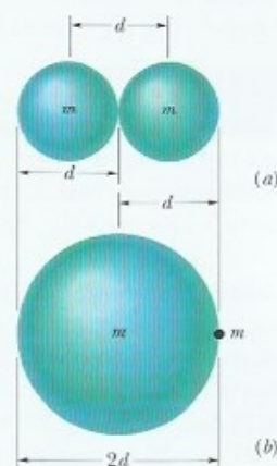
Figura 19-6 (a) Uma colisão acontece quando os centros de duas moléculas ficam a uma distância d , onde d é o diâmetro das moléculas. (b) Uma representação equivalente, porém mais conveniente, é pensar na molécula em movimento como tendo um raio d e em todas as outras moléculas como pontos. A condição para que aconteça uma colisão permanece a mesma.
