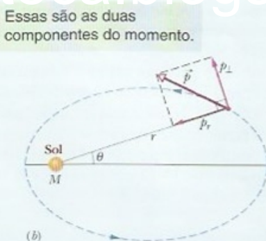
Figura 13-13 (a) No instante \Delta t , o segmento de reta r que liga o planeta ao Sol se desloca de um ângulo \Delta\theta , varrendo uma área \Delta A (sombreada). (b) O momento linear \vec{p} do planeta e suas componentes.
