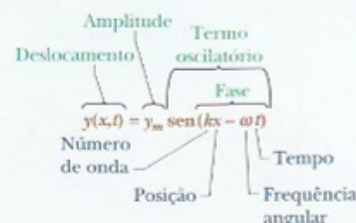
Figura 16-3 Nomes das grandezas da Eq. 16-2, para uma onda senoidal transversal.
