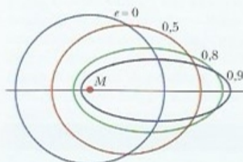
Figura 13-15 Quatro órbitas com diferentes excentricidades e em torno de um corpo de massa M . As quatro órbitas têm o mesmo semieixo maior a e, portanto, a mesma energia mecânica total E .
