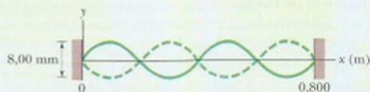
Figura 16-22 Oscilações ressonantes em uma corda sob tensão.
