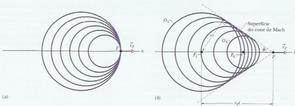
Figura 17-22 (a) Uma fonte sonora F se move com uma velocidade v_F igual à velocidade do som v , e, portanto, com a mesma velocidade que as frentes de onda que produz. (b) Uma fonte F se move com uma velocidade v_F maior que a velocidade do som, e, portanto, mais depressa que as frentes de onda. Quando a fonte estava na posição F_1 , produziu a frente de onda O_1 ; quando estava na posição F_0 , produziu a frente de onda O_0 ; e da sua posição atual F , produz a frente de onda O . As frentes de onda esféricas se espalham com a velocidade do som v e se superpoem na superfície de um cone conhecido como cone de Mach, formando uma onda de choque. A superfície do cone possui um semiângulo \theta e é tangente a todas as frentes de onda.
