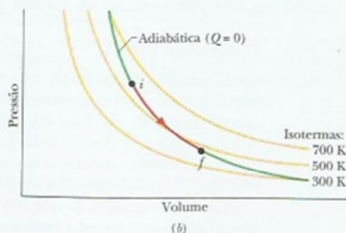
Figura 19-15 (a) O volume de um gás ideal é aumentado reduzindo o peso aplicado ao êmbolo. O processo é adiabático ( Q = 0 ). (b) O processo se desenvolve de i para f ao longo de uma adiabática no diagrama p - V .
