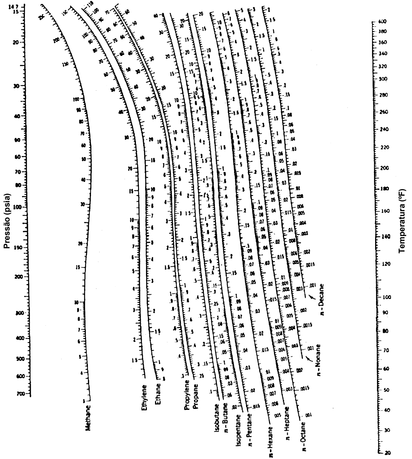
Nomógrafo de "DePriester"
