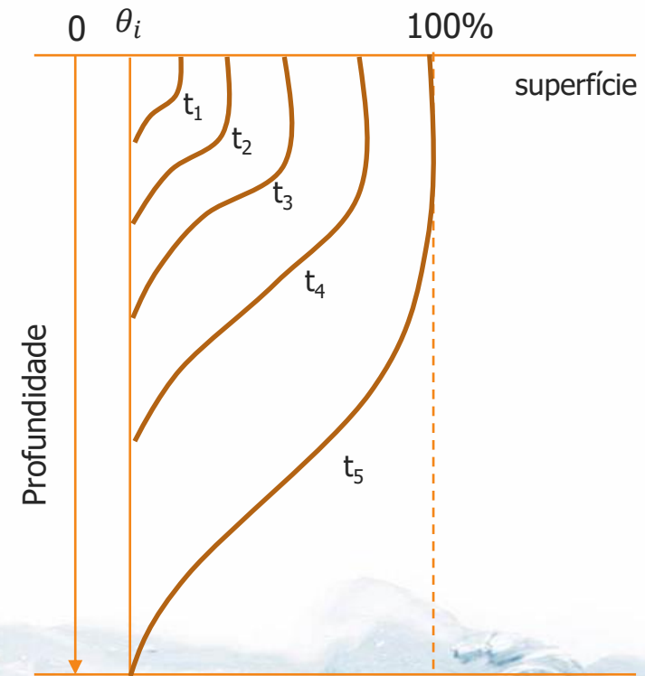
Mudança do perfil de umidade com o tempo
