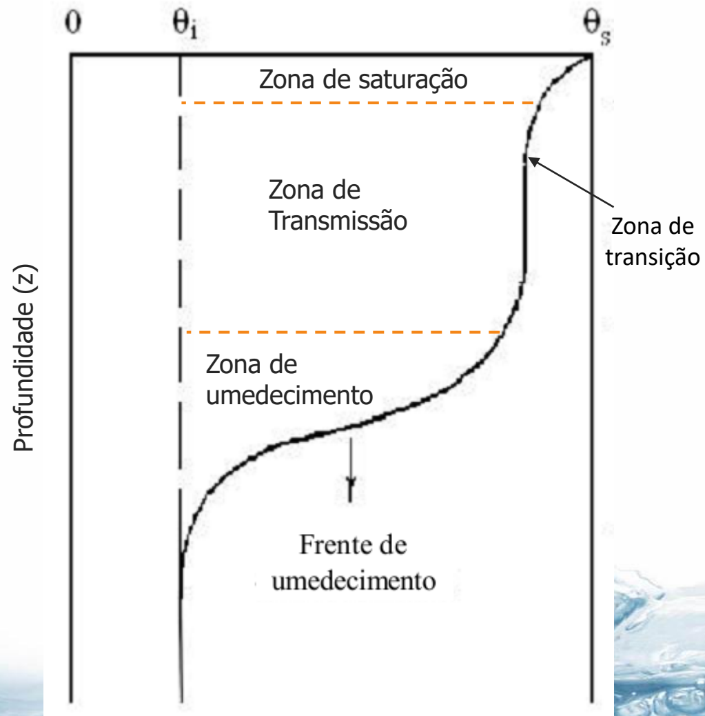
Mudança do perfil de umidade com o tempo
