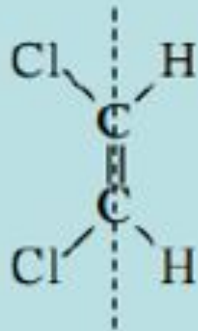
Cis-1,2-dicloroeteno
