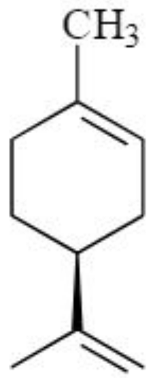
S-limoneno
