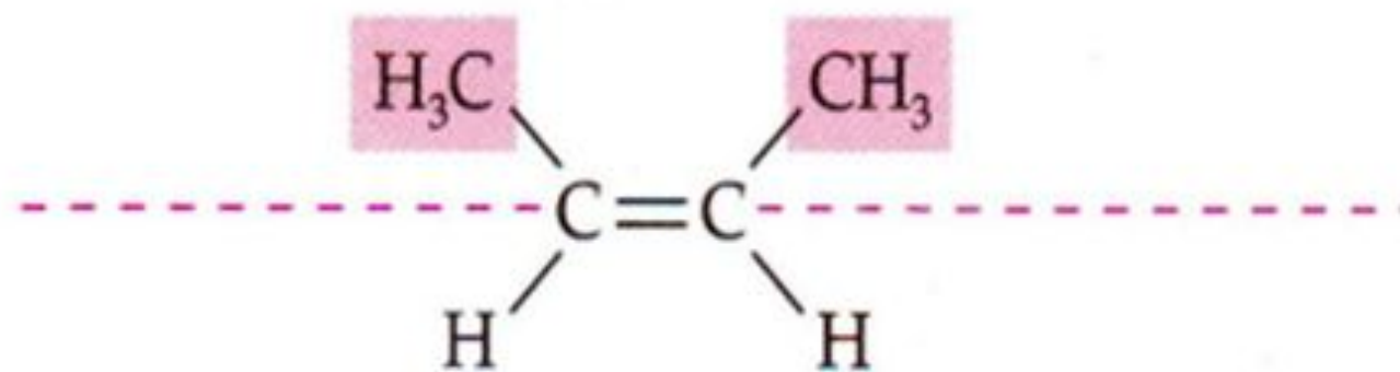
cis-but-2-eno
