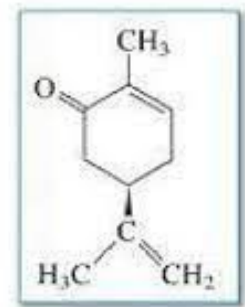
(R)-(-)-Carvona (do óleo de hortelã)
