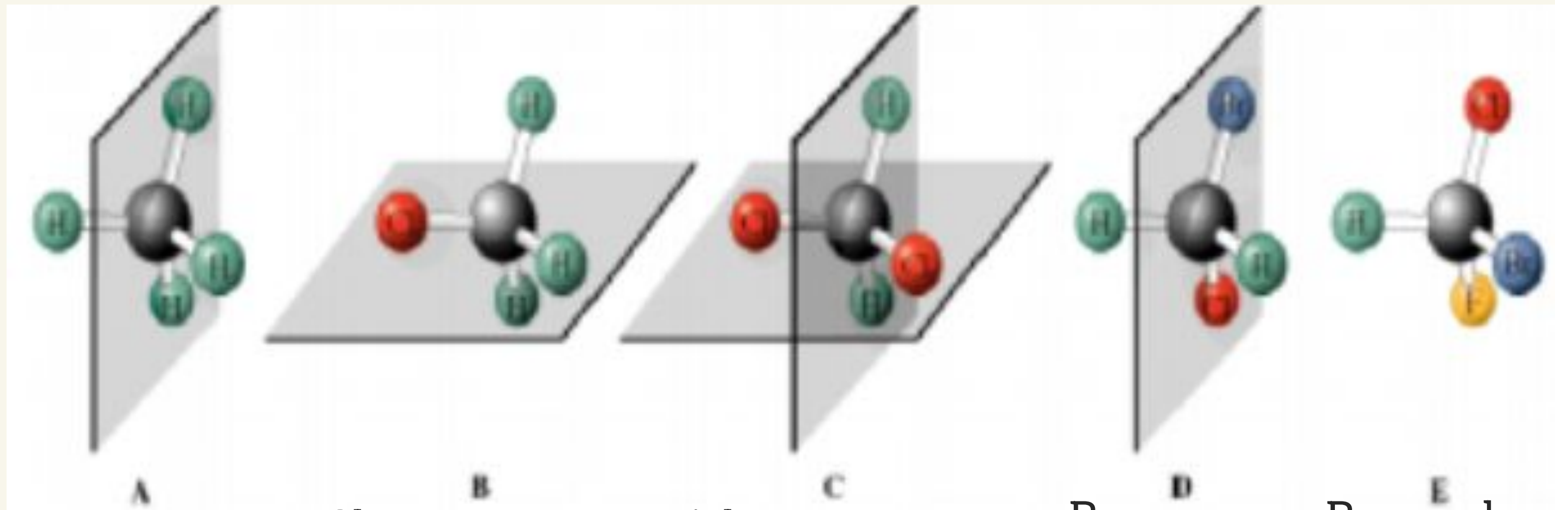
Metano
