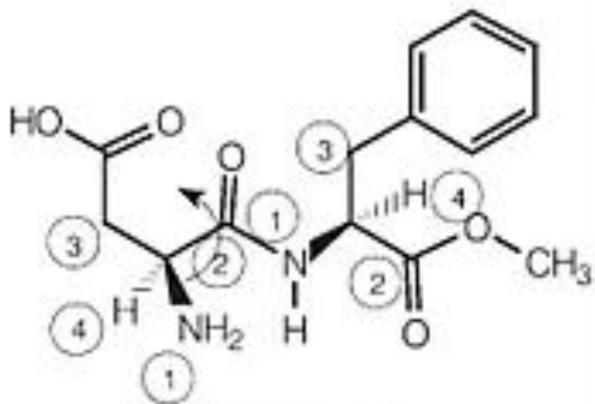
(S,S)-Aspartamo sabor doce
