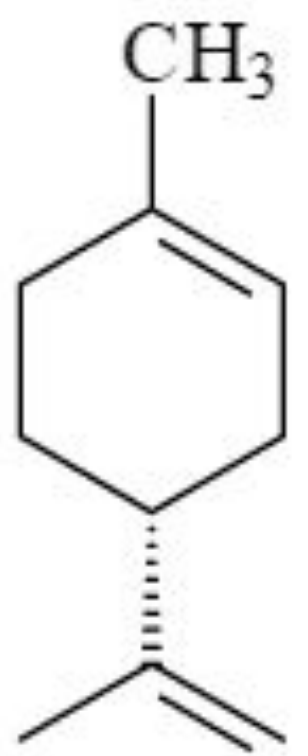
R-limoneno
