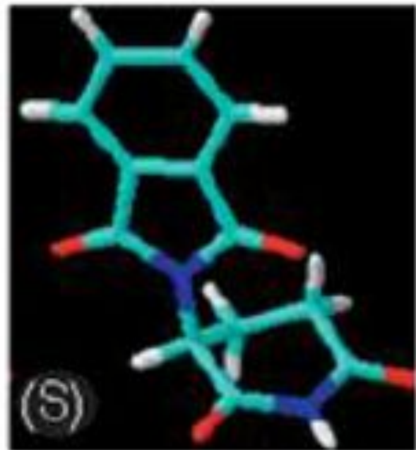
(S)-Talidomida teratogênico
