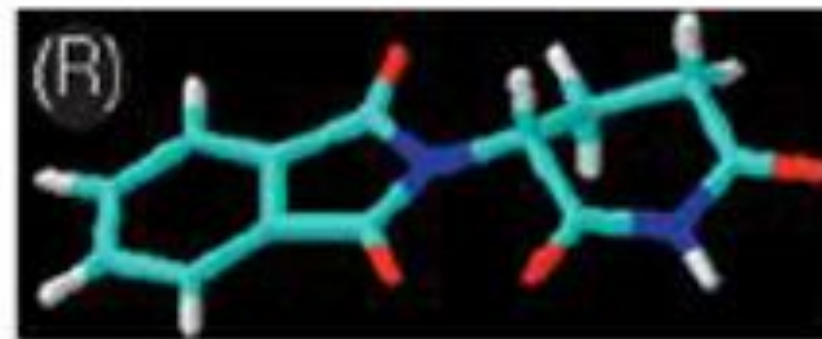
(R)-Talidomida sedativo
