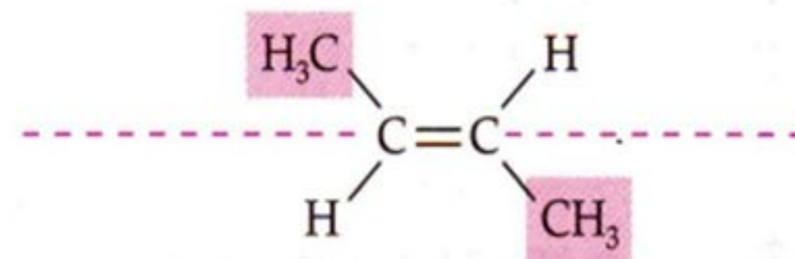
trans-but-2-eno
