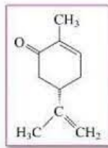
(S)-(+)-Carvona (do óleo da semente de alcaravia)
