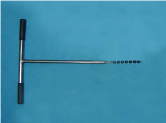
Fig. 10. Trado de rosca tipo Mathieson para a instalação de tensiômetros.
