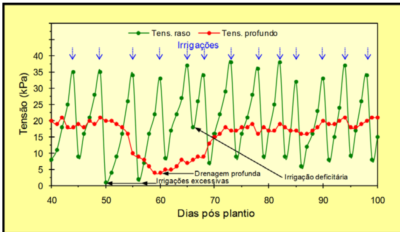
Fig. 15. Valores médios das leituras de tensiômetros, de três estações de controle, instalados a 50% e 100% da profundidade efetiva do sistema radicular de uma cultura de melancia, ao longo de um período do ciclo de desenvolvimento das plantas, com indicativo dos momentos das irrigações.
