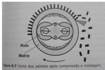
Figura 9.7 Corte dos p elletes ap os compress o e moldagem.
