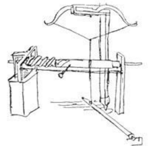
Esboço de um torno de pedal e duplo polo de Leonardo da Vinci, que não conseguiu construir devido à falta de meios (século XV)
