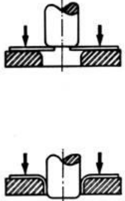
Flangeamento
