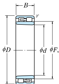
Tipo NNU Furo Côncavo
