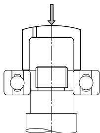
Fig. 14.1 Prensação do Anel Interno
