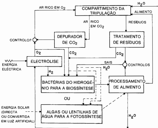
Figura 20-5. Diagrama simplificado de um sistema de bio-reciclagem de materiais baseado em bactérias quimiossintéticas ou em plantas fotossintéticas.
