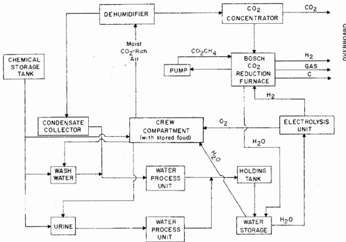
Figura 20-4. Diagrama simplificado da teoria de um sistema mecânico-químico de reciclagem de materiais. Veja-se na Figura 20-3 um modelo em funcionamento.
