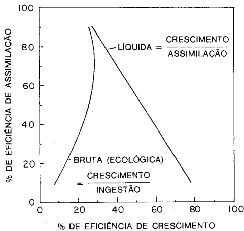
Fig. 3-13. Relações entre eficiência de crescimento de tecido, eficiência de crescimento ecológico e eficiência de assimilação em populações animais. (Segundo Welch, 1968.)
