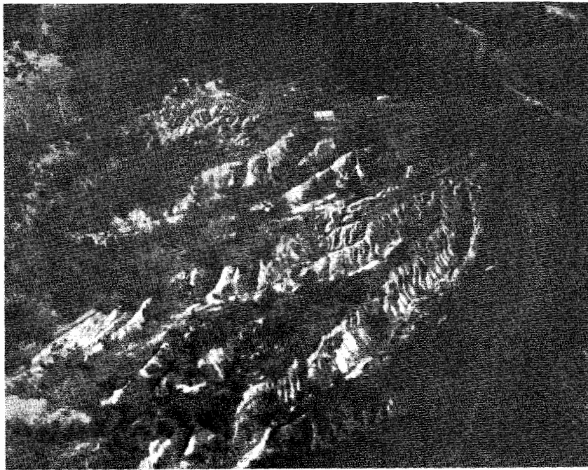
Figura 2-8. A. A Copper Basin em Copperhill, Tennessee, sugere como seria a terra sem vida. Uma floresta luxuriante cobria esta área até os vapores de umas fundições terem exterminado toda a vegetação. Se bem que os métodos modernos de preparação dos minérios já não emitam vapores, a vegetação não se restabeleceu. (Fotografia dos U.S. Forest Service.) B. Terra de cultura no Mississippi arruinada pela erosão. Tais abusos deixam ao abandono casas e gente pobre. (Fotografia dos U.S. Forest Service.)
