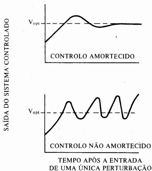
Figura 10-2. Um sistema básico de retroação tal como é concebido na teoria do controlo (adaptado de Waterman, 1968). Um valor de referência do estado ou taxa de saída do sistema controlado, V_{opt} , é comparado, através de um mecanismo (o comparador), com o presente valor do sistema, V_{saida} . A diferença é um erro, e , que é utilizado pelo mecanismo de controlo para proporcionar uma taxa de entrada modificada, r , para o sistema controlado. O valor de referência poderá ser, ele próprio, uma função de V_{saida} .
