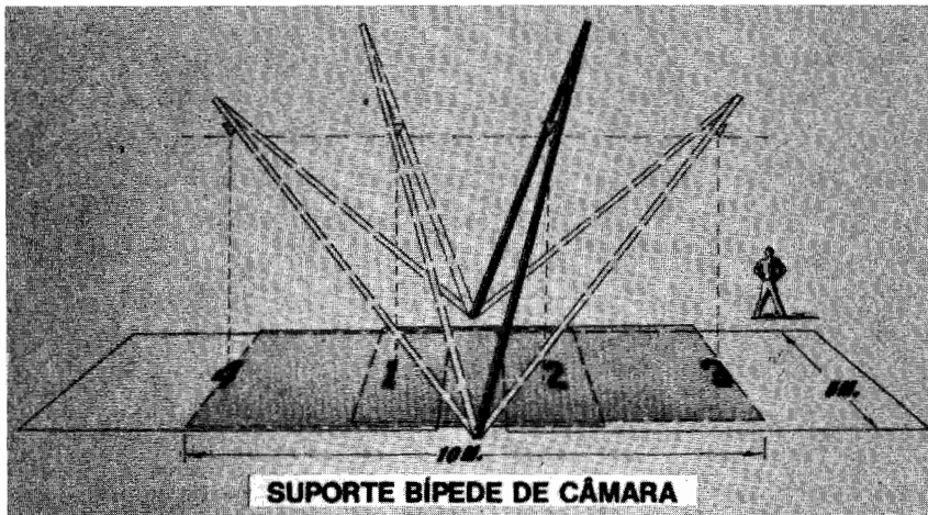
Figura 18-5. Suporte bípede de câmara utilizado na estereofotografia fotogramétrica para obtenção de fotografias estereoscópicas da área sombreada. A câmara está suspensa verticalmente no triângulo e oscila-se o bípede para as posições precisas indicadas. Um dispositivo portátil deste tipo pode ser montado e erguido por dois homens. (Modificado de Whittlesey, 1966.)
