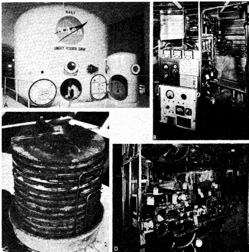
Figura 20-3. Um «Sistema Integrado de Sustentação da Vida» simulado que recicla água e gases por meios mecânicos e químicos. A. Vista exterior da câmara de sustentação da vida. A pequena câmara lateral, à direita, é a câmara sob pressão por onde os astronautas entram e saem. B. Equipamento de reciclagem atmosférica. C. Fotografia das placas catalizadoras de redução do \text{CO}_2 de Bosch, mostrando carbono acumulado que deve ser expelido da cápsula. D. Controlos de administração da água com tanques de armazenamento em cima e em baixo. As imagens B e D ilustram de forma impressionante quanto material de «engenharia» complicado é preciso para substituir as mais elementares funções da natureza! (Fotografias reproduzidas por cortesia do Langley Research Center, Langley, Virgínia.)
