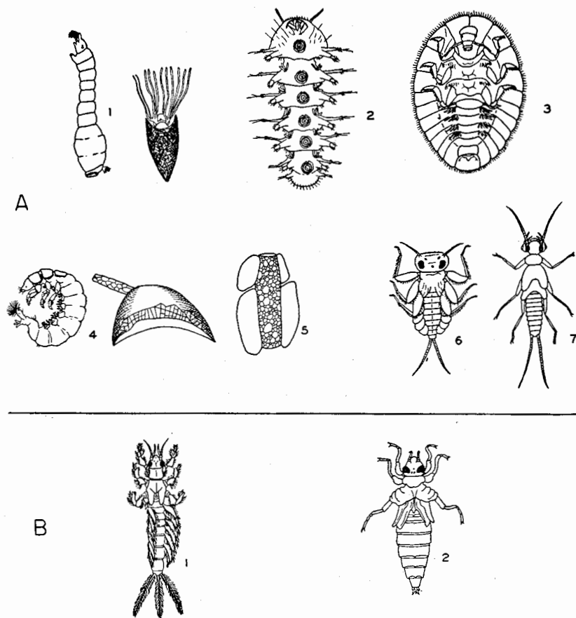
Figura 11-12. Alguns animais característicos de cursos de água. A. Gêneros representativos das comunidades de rápidos, ilustrando várias adaptações à vida em correntes rápidas. Este grupo é muitas vezes chamado, apropriadamente, «fauna torrencial». 1. Uma larva de pequena mosca de gado, Simulium (Simuliidae) e a sua pupa (à direita) num casulo fixo à rocha; repare-se na ventosa existente na extremidade posterior da larva e nos «leques» existentes na cabeça, com os quais apanha alimento da água. 2. Uma larva de blefarocerídeo, Bibiocephala (note-se a fiada de ventosas ventrais). 3. Uma «moeda da água», Psephenus , a larva de um coleóptero dos rápidos (Psephenidae). 4. Uma larva de tricóptero, Hydropsyche e a rede que tece (a abertura fica voltada para a corrente), com o respectivo abrigo. 5. O casulo de um tricóptero, Goera , com pedrinhas aderentes, que servem de lastro. 6. Uma ninfa de efemeróptero, Iron , e 7, uma ninfa de plecóptero, Isogenus , ambas com corpos achatados e linhas favoráveis à corrente, adaptadas para se agarrarem à face inferior das pedras. (Nota: a maioria das ninfas de plecópteros apresentam duas «caudas» e a maioria das ninfas de efemerópteros três, como se vê em B-1. Iron é atípica a este respeito). B. Dois tipos que escavam galerias e vivem nas margens da corrente ou no fundo dos pegos. 1. Uma ninfa mineira de efemeróptero, Hexagenia . 2. Uma ninfa mineira de tira-olhos, Progomphus (Reproduzido de Robert W. Pennak, «Fresh-water Invertebrates of the United States», 1953, The Ronald Press Company.)
