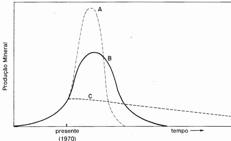
Figura 15-1. Modelos alternativos de esgotamento para os recursos minerais. A. Modelo de extração e esgotamento rápidos de minerais (ou outras matérias-primas não renováveis) que terá lugar desde que se insista na prática actual de remoção, uso e desperdício. Alguns metais básicos ficarão «esgotados» antes do ano 2000, caso se mantenha este modelo. B. O tempo de esgotamento pode ser prolongado mediante reciclagem parcial e menor esbanjamento na utilização. C. Uma reciclagem eficiente, combinada com conservação e substituições apertadas (utilizando quanto possível material alternativo mais abundante), pode estender as curvas de esgotamento indefinidamente. (Diagrama adaptado de Cloud, 1969.)
