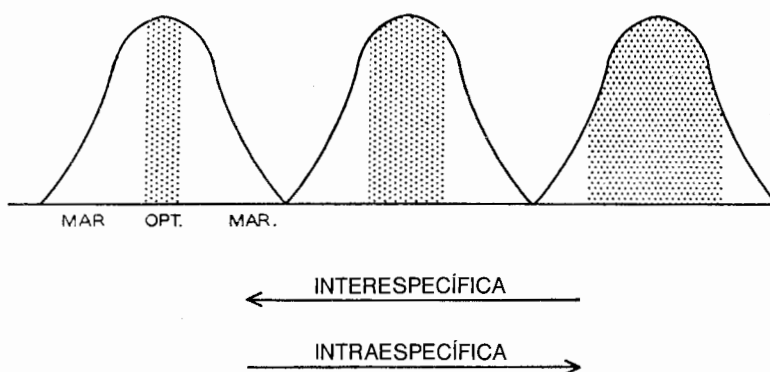
Figura 7-31. O efeito da competição na distribuição do habitat de aves. Quando a competição intraespecífica domina, as espécies estendem-se e ocupam áreas menos favoráveis (marginais); onde a competição interespecífica é intensa, as espécies tendem a ficar restringidas a um âmbito mais estreito que integra as condições óptimas. (Adaptado de Svardson, 1949.)
