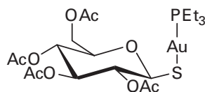
68 Auranofin
