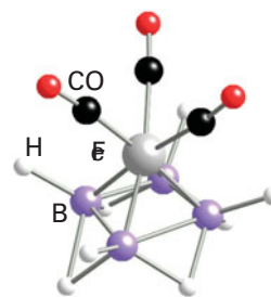
32 [Fe(CO)_3B_4H_8]
