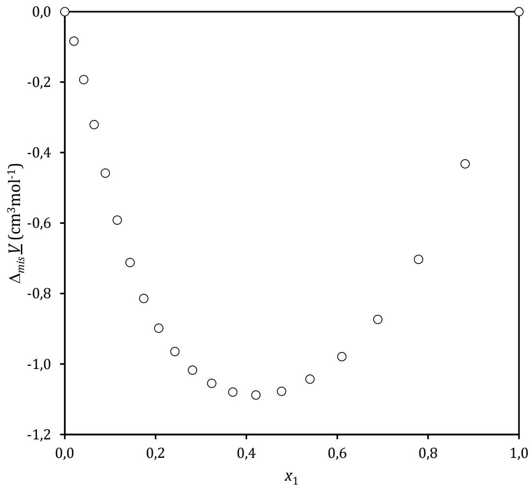
Figura 1. Variação de volume devida à mistura para o par etanol (1) e água em fase líquida a 298,15 K e pressão atmosférica.
