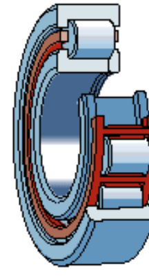
NUP
