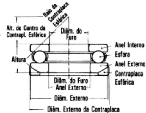
Rolamento Axial de Esferas de Escora Simples
